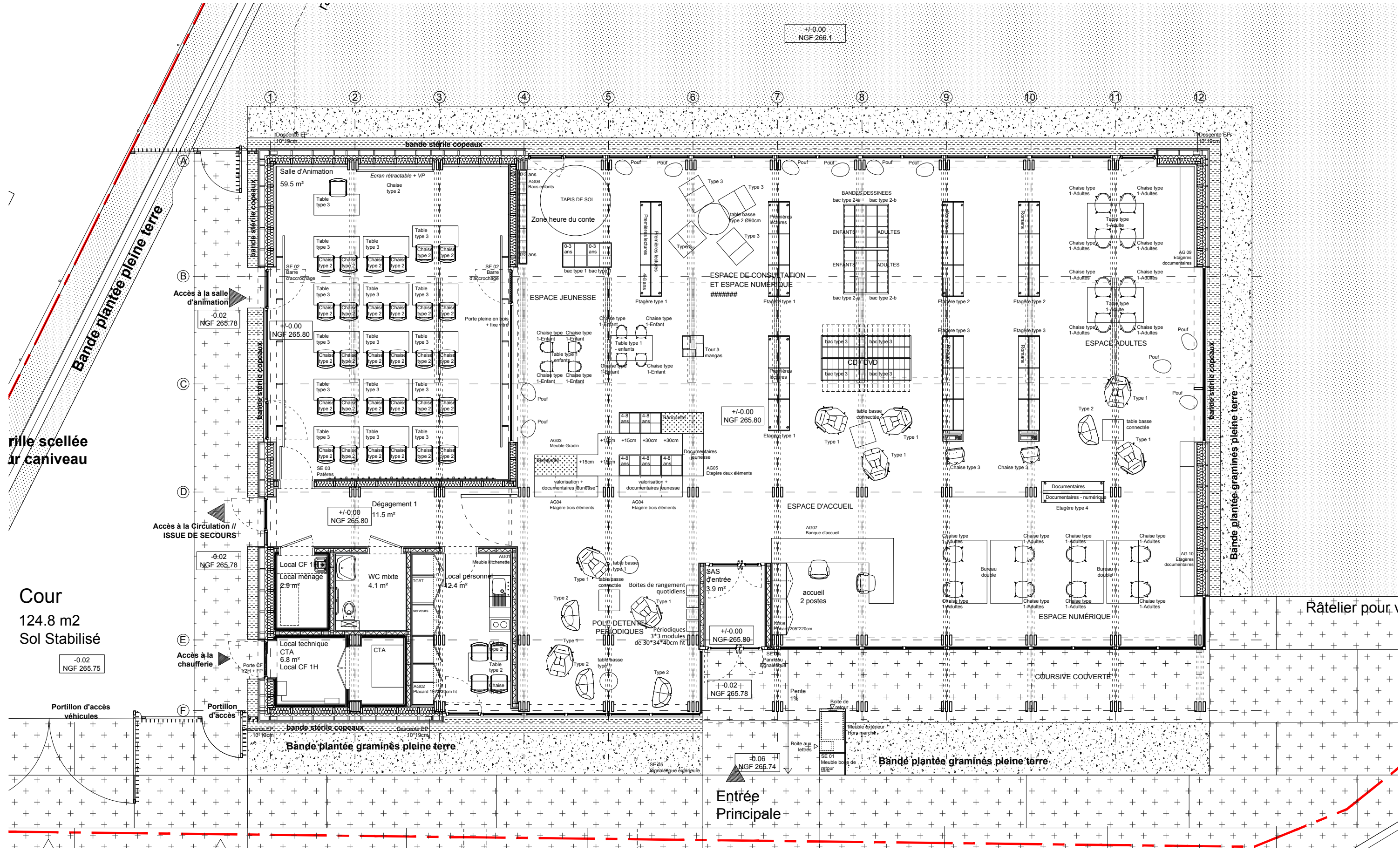
PLAN DE MOBILIER echelle 1/100eme
