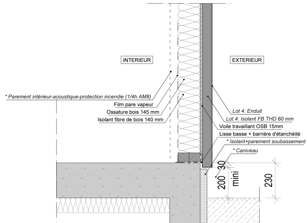
Détail : principe de composition des façades
