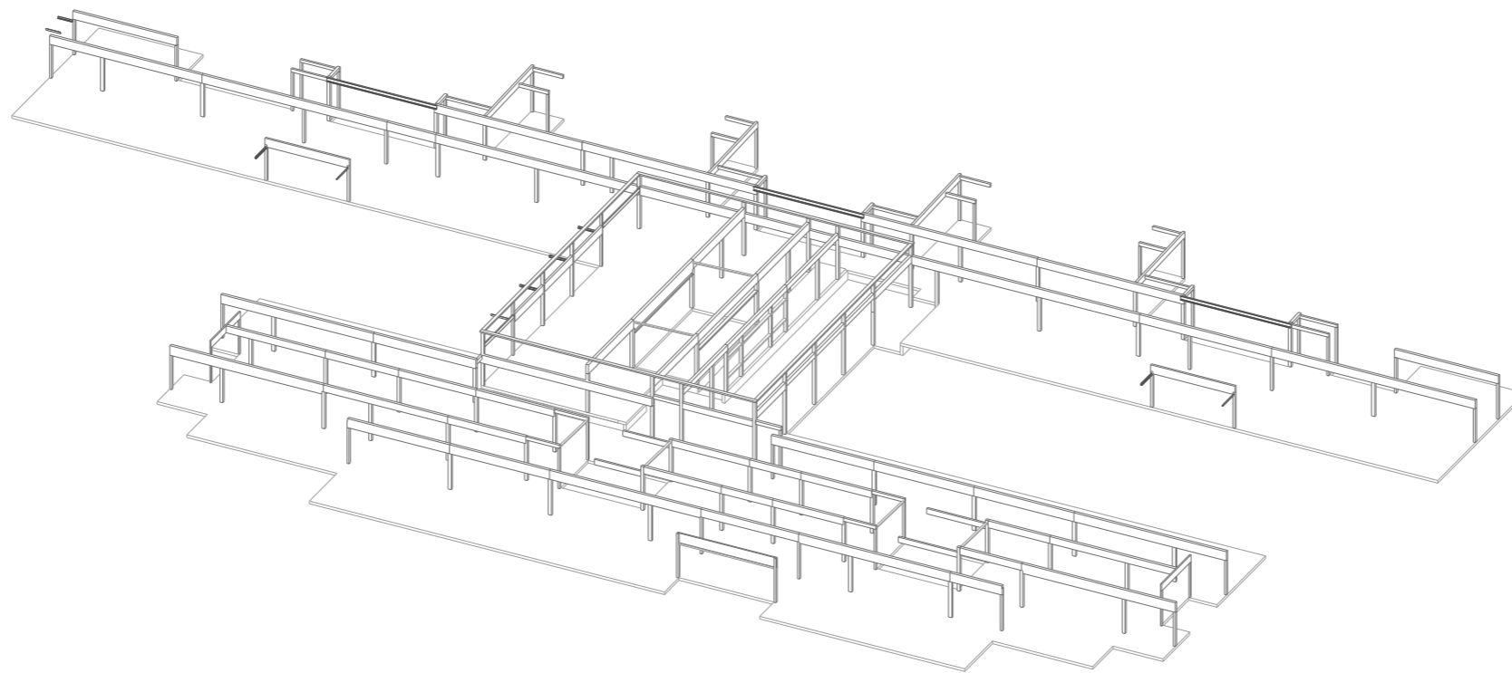
Axonométrie partielle : structure principale
