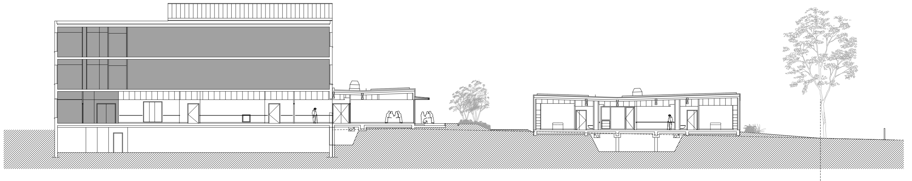
coupe longitudinale
