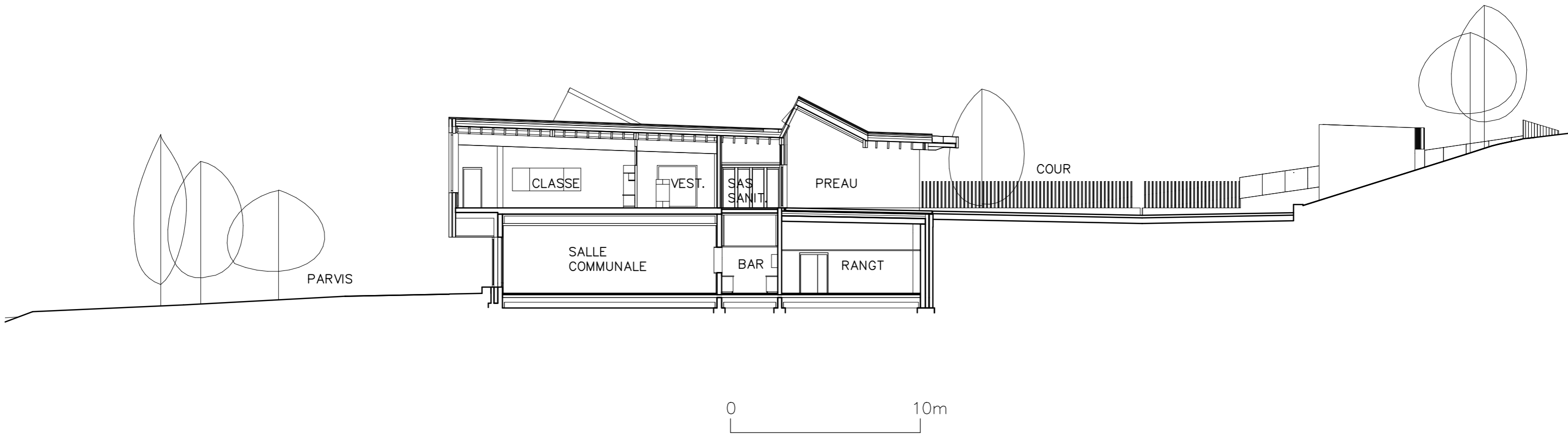
COUPE TRANSVERSALE ECHELLE: 1/200 GROUPE SCOLAIRE ET SALLE COMMUNALE A ALEX
