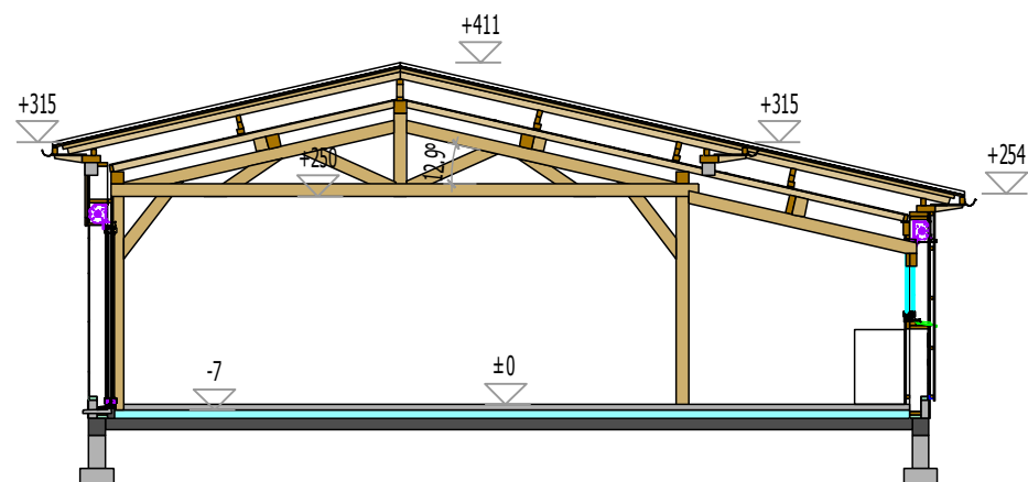
COUPE B.B
