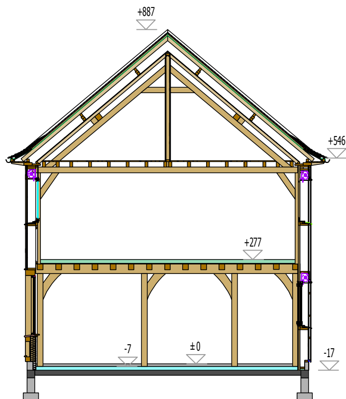
COUPE C.C
