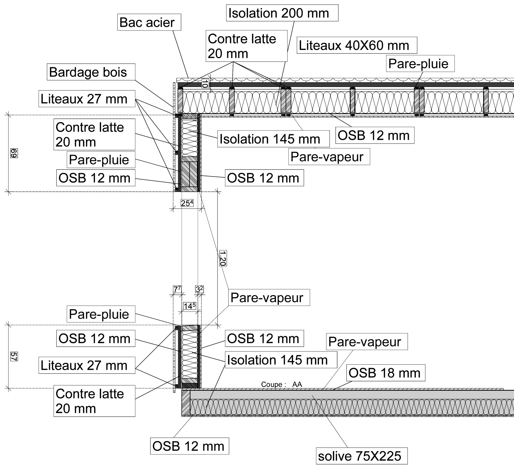
COUPE PLONGITUDINALE
