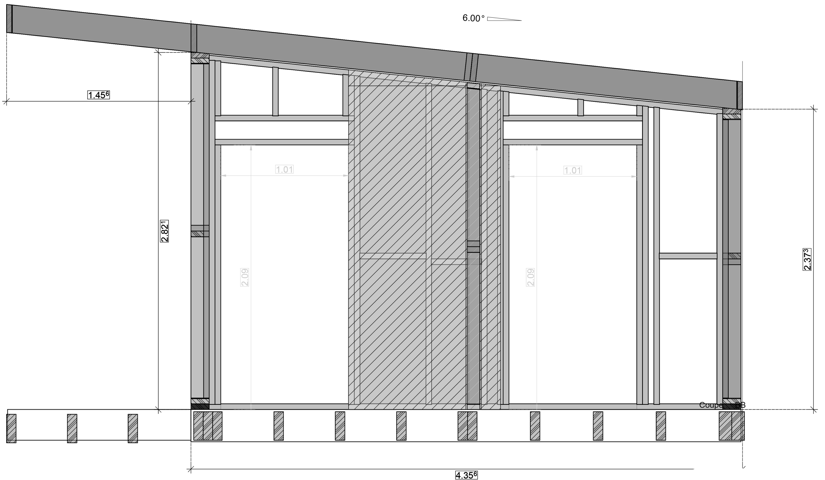
COUPE TRANSVERSALE
