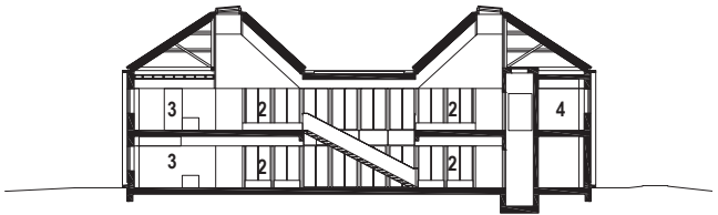
Coupe BB
