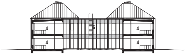
Coupe AA
