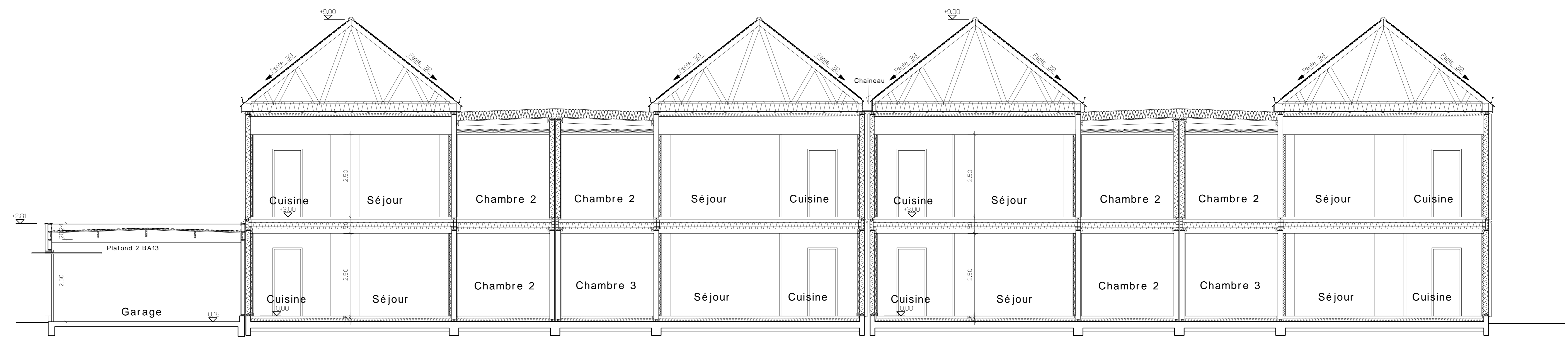
Bâtiments A et B Coupe AA
