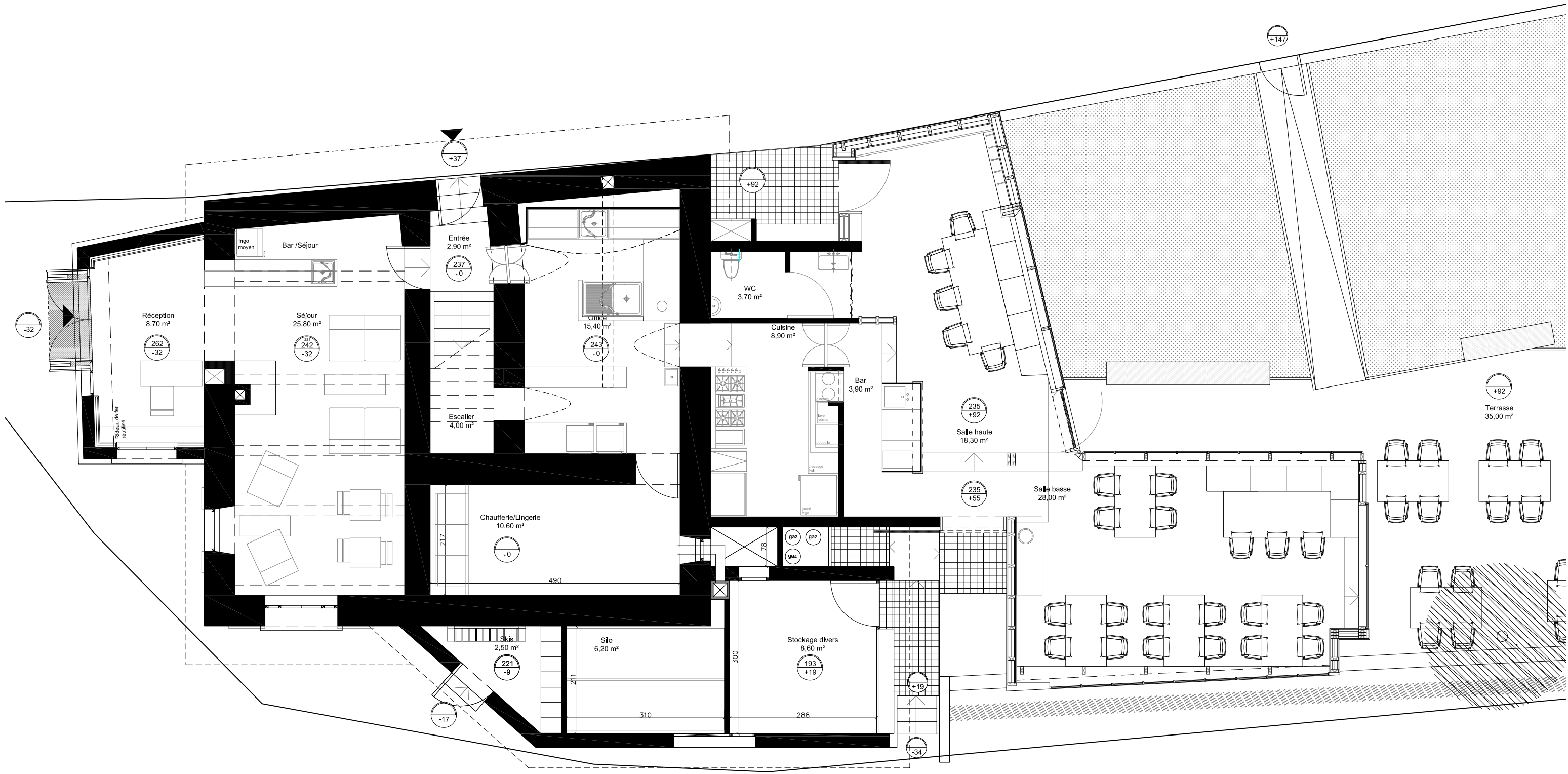
PLAN RDC | 1:75
