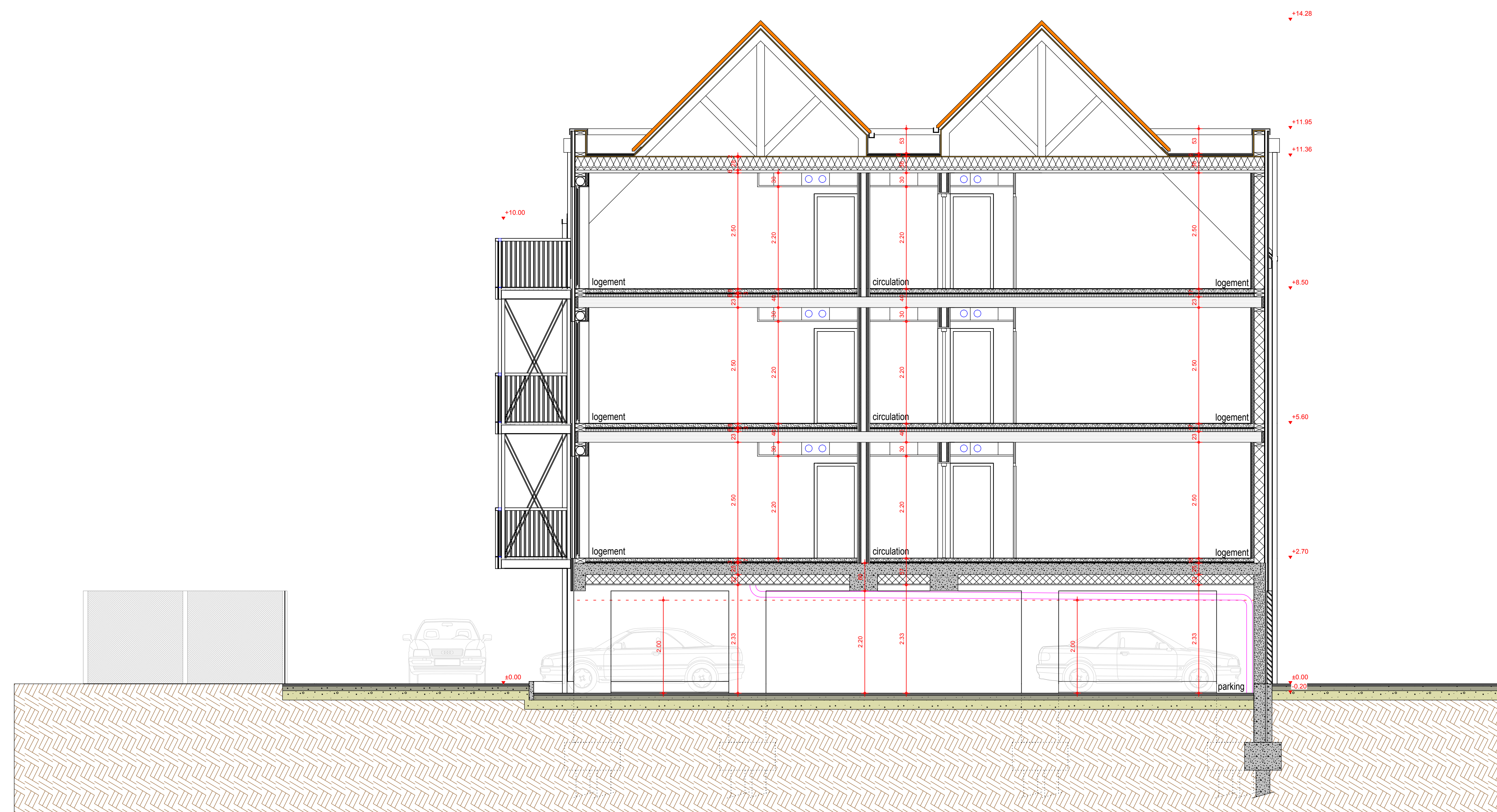
COUPE A-A ech : 1/50ème
