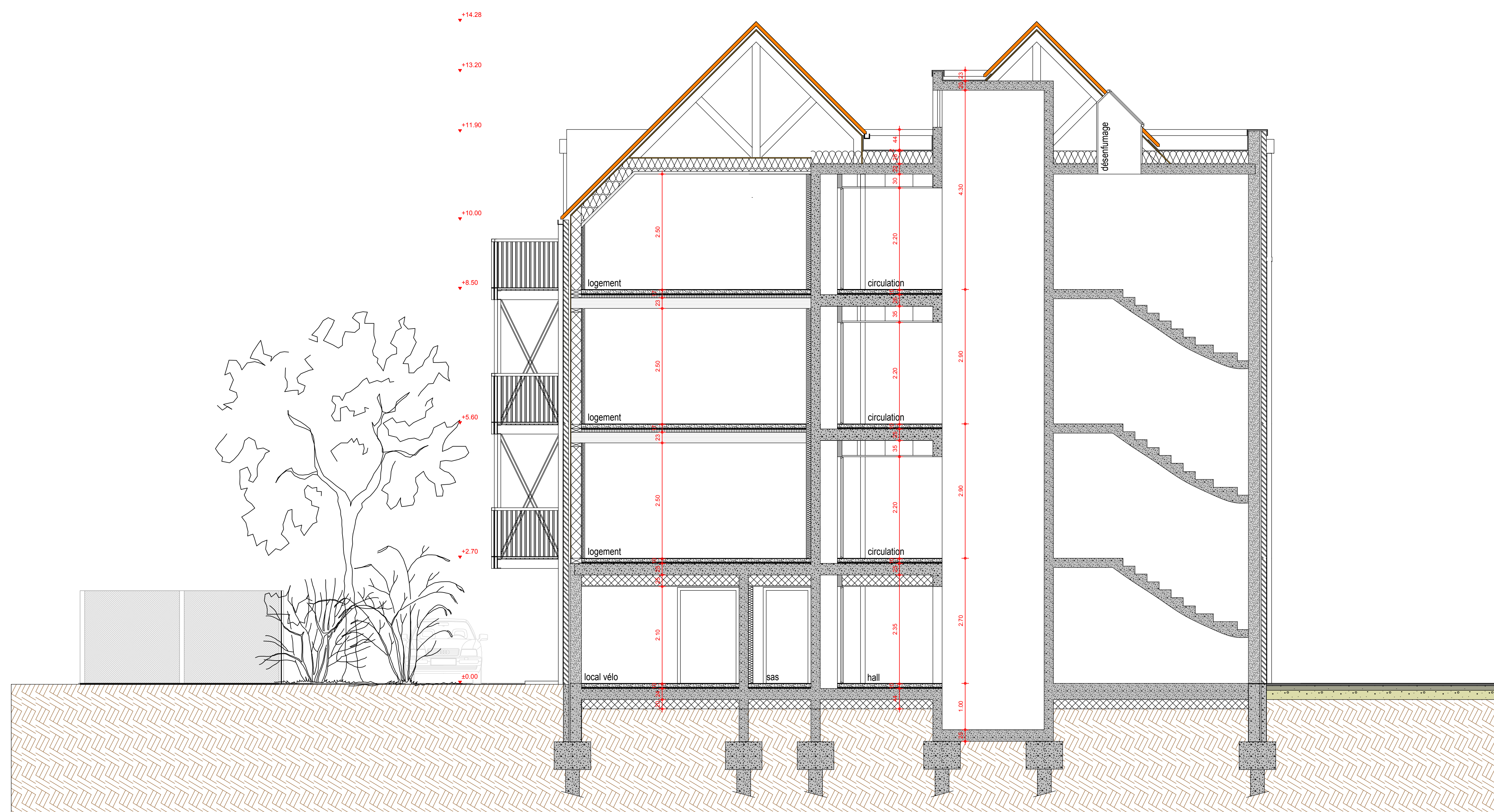
COUPE B-B ech : 1/50ème
