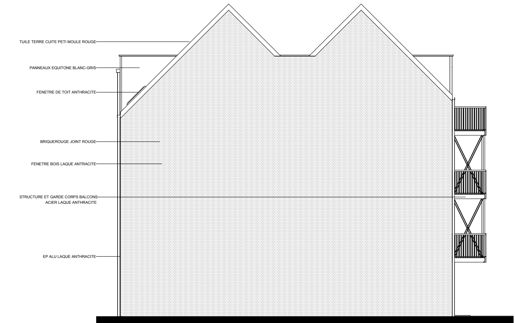
ELEVATION PIGNON OUEST ech 1/100 ème
