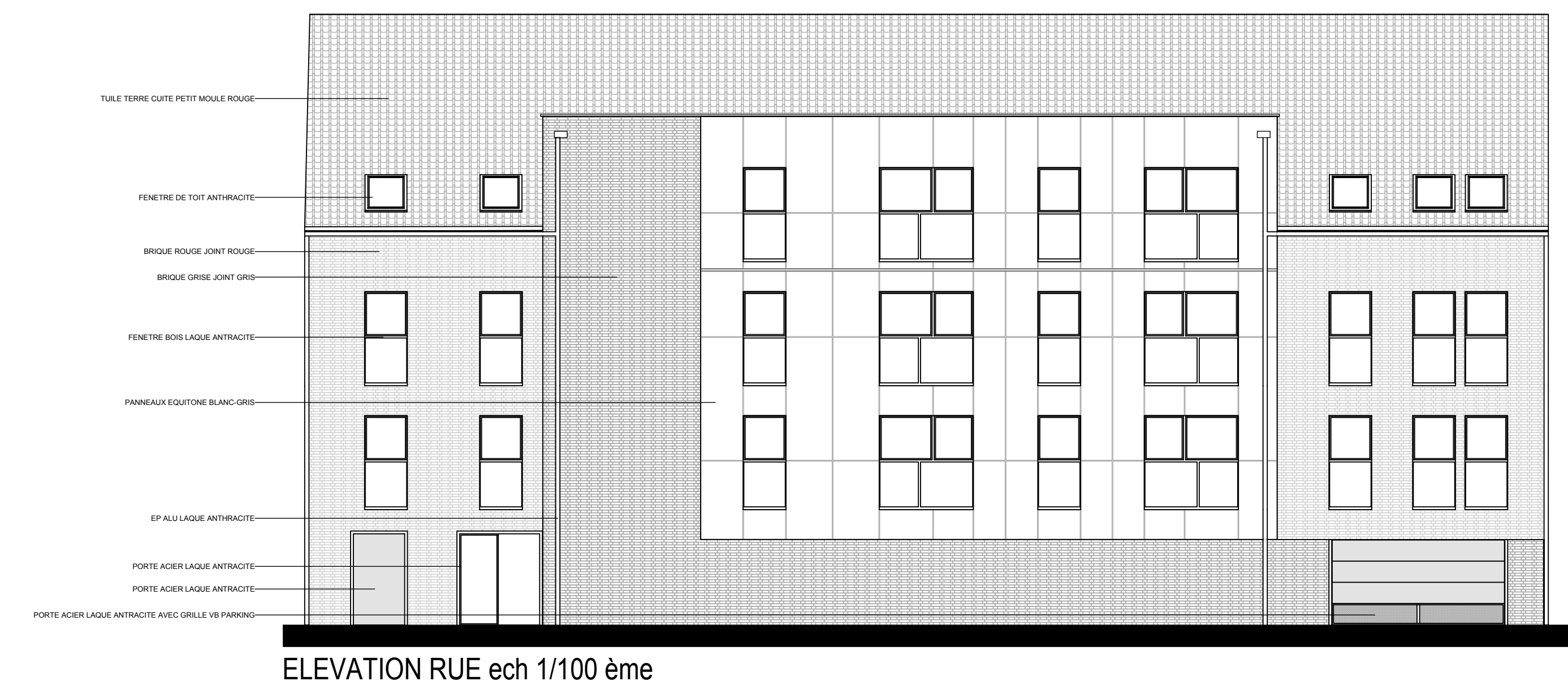
ELEVATION RUE ech 1/100 ème
