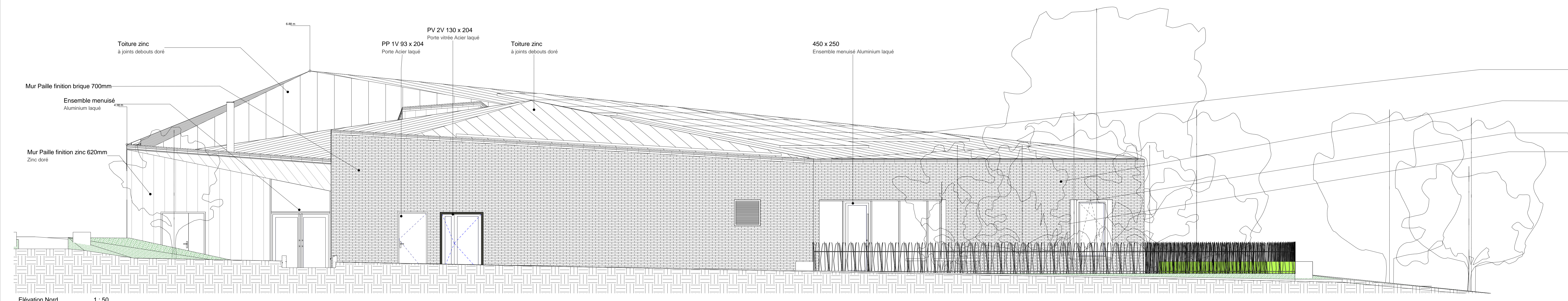
Elevation Nord 1 : 50
