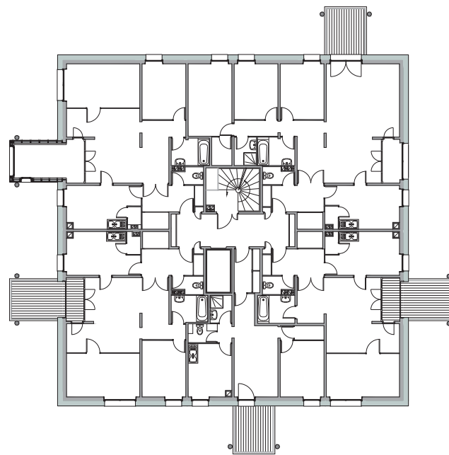
PLAN DU R+6
