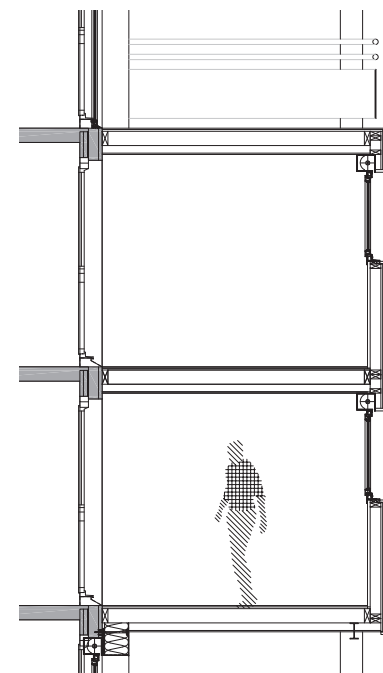
DÉTAIL STRUCTUREL D'ORIEL
