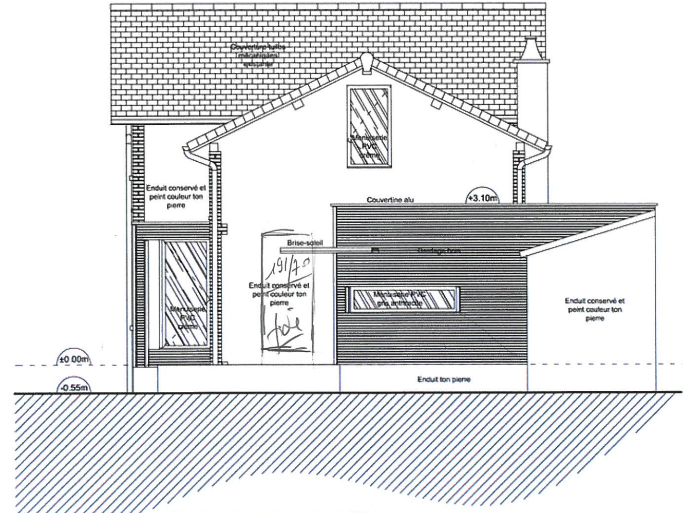
Elévation Nord-Est - Ech. : 1/75
