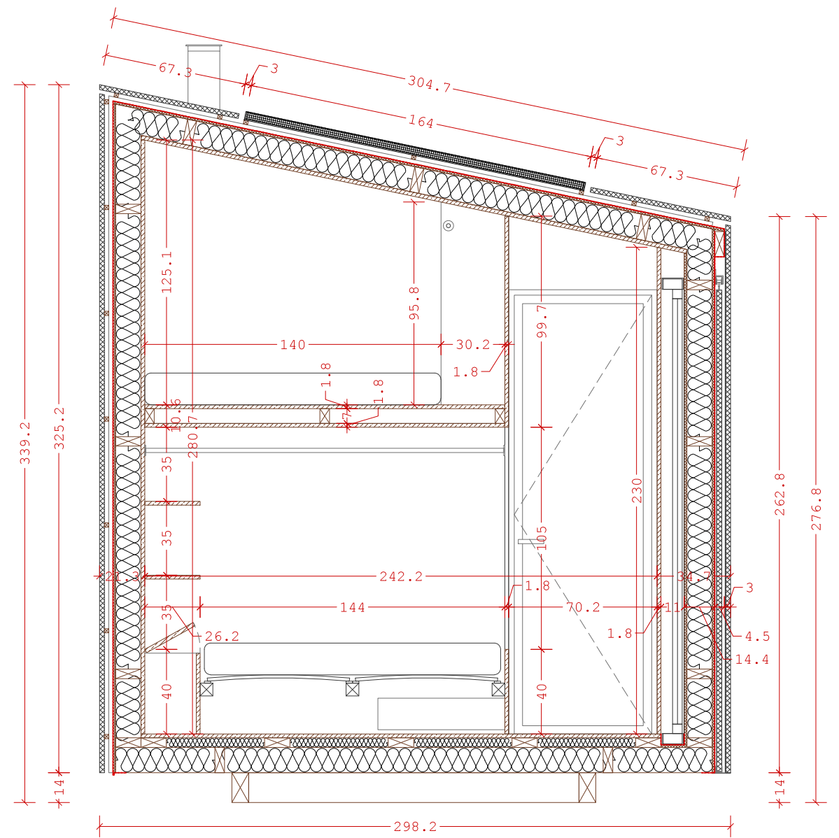
COUPE 2
