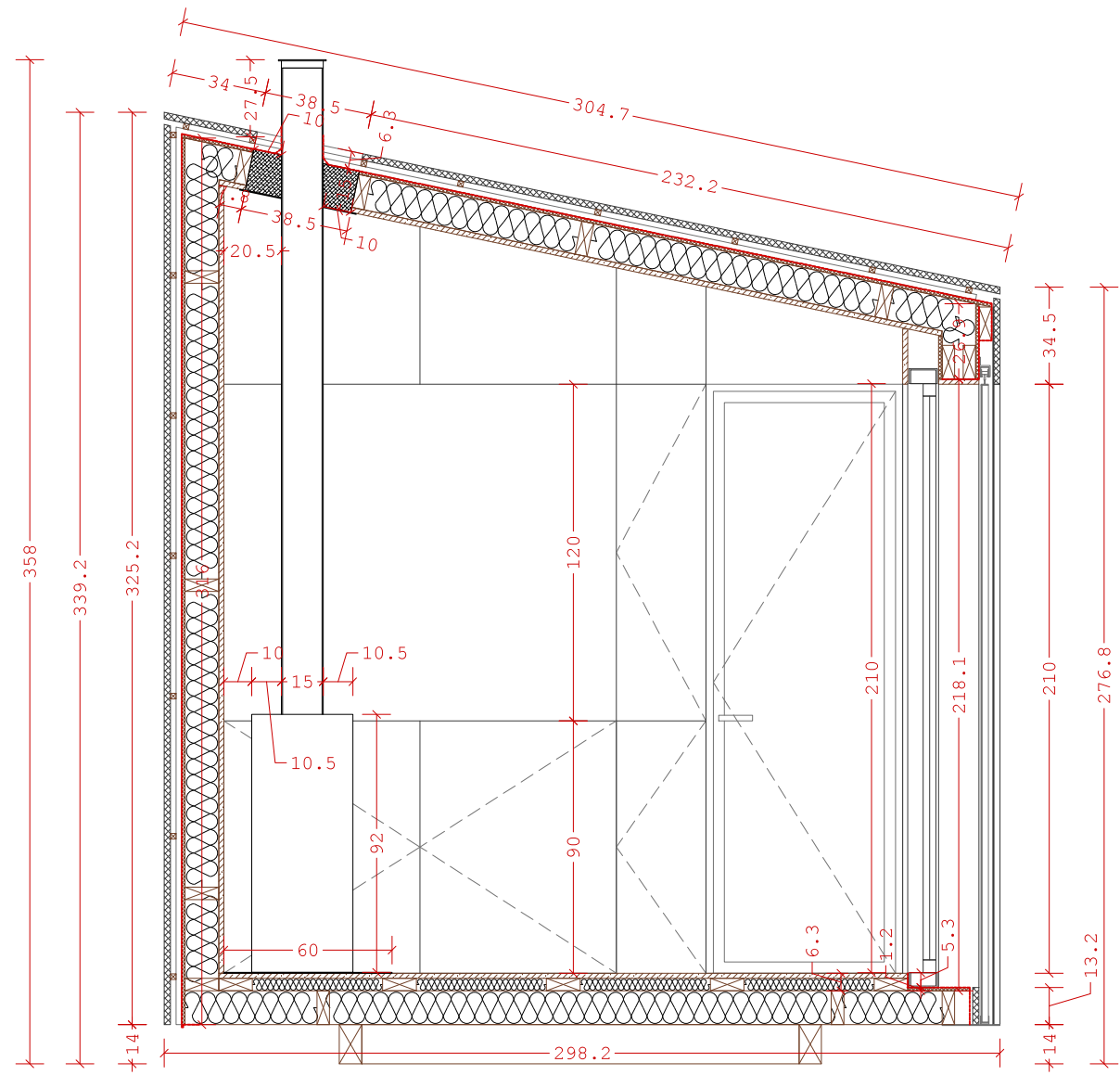
COUPE 1
