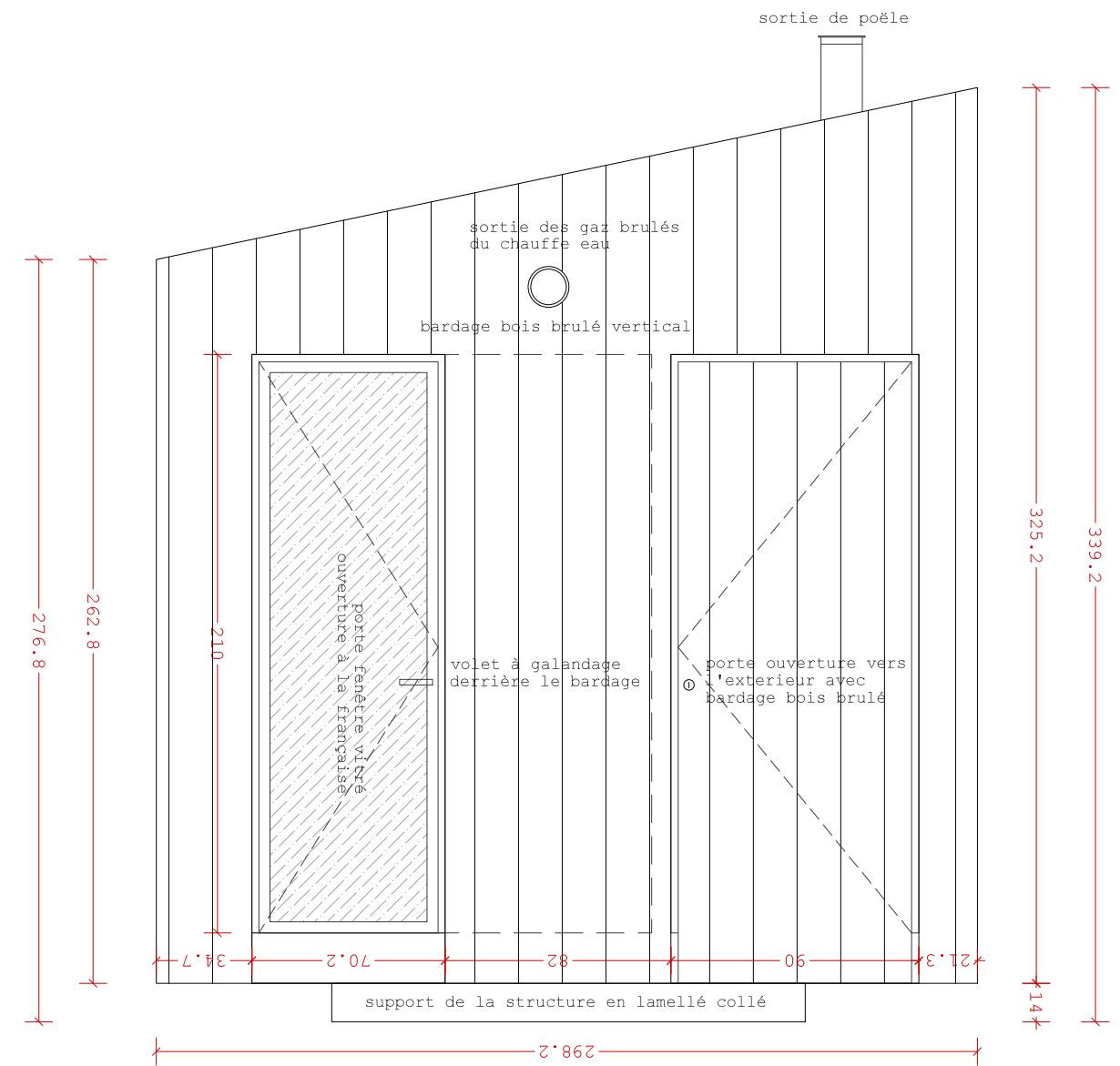
FACADE EST
