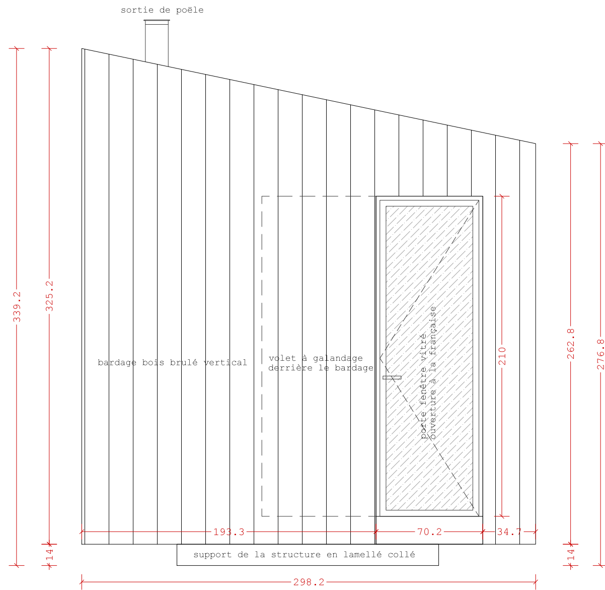
FACADE OUEST
