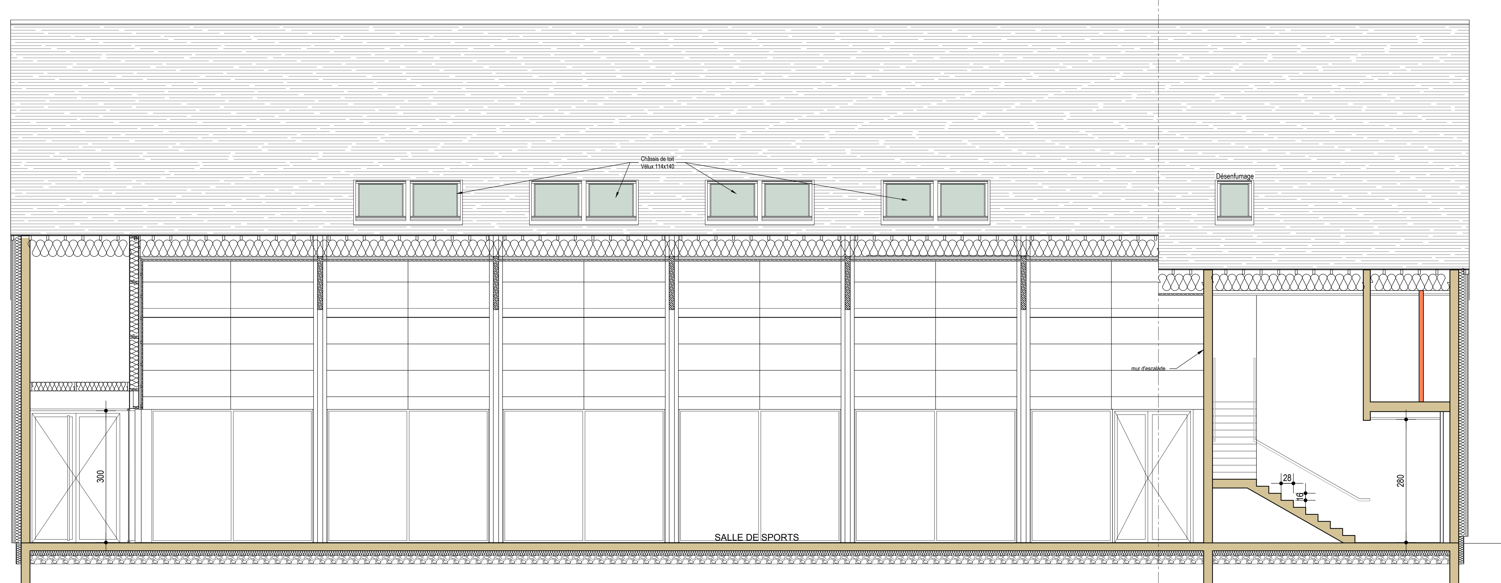
COUPE 5.5
