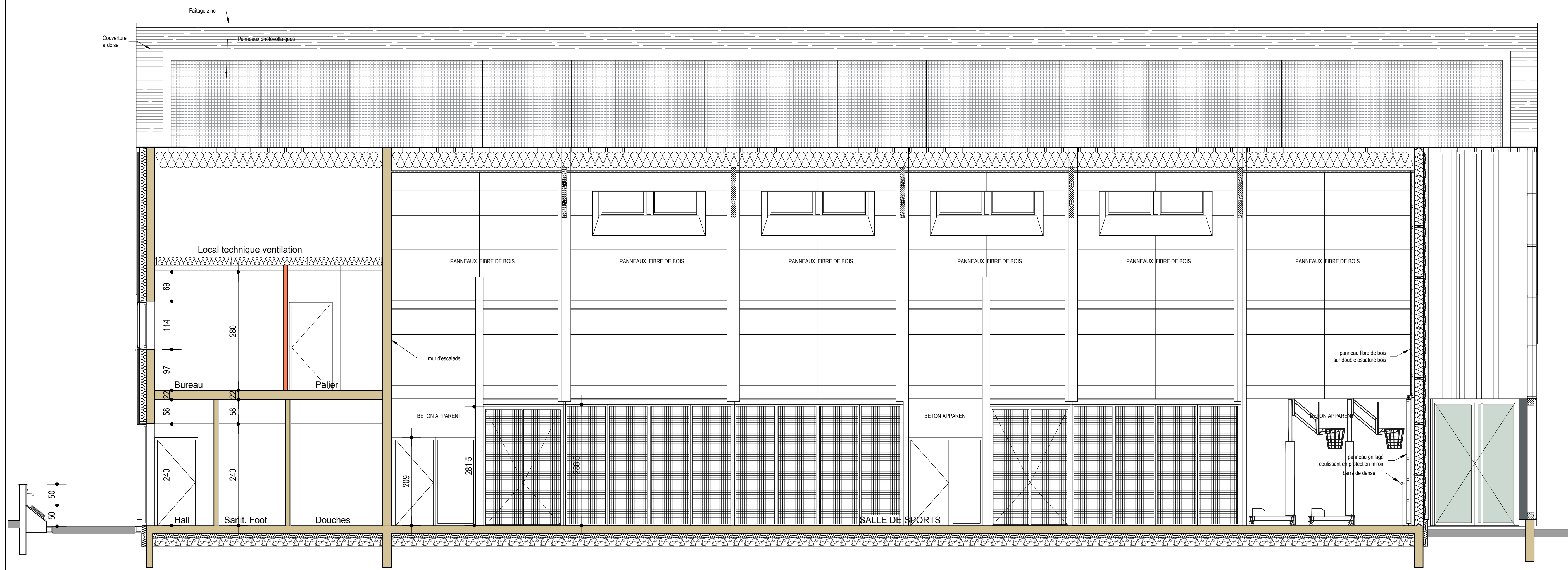
COUPE 4.4
