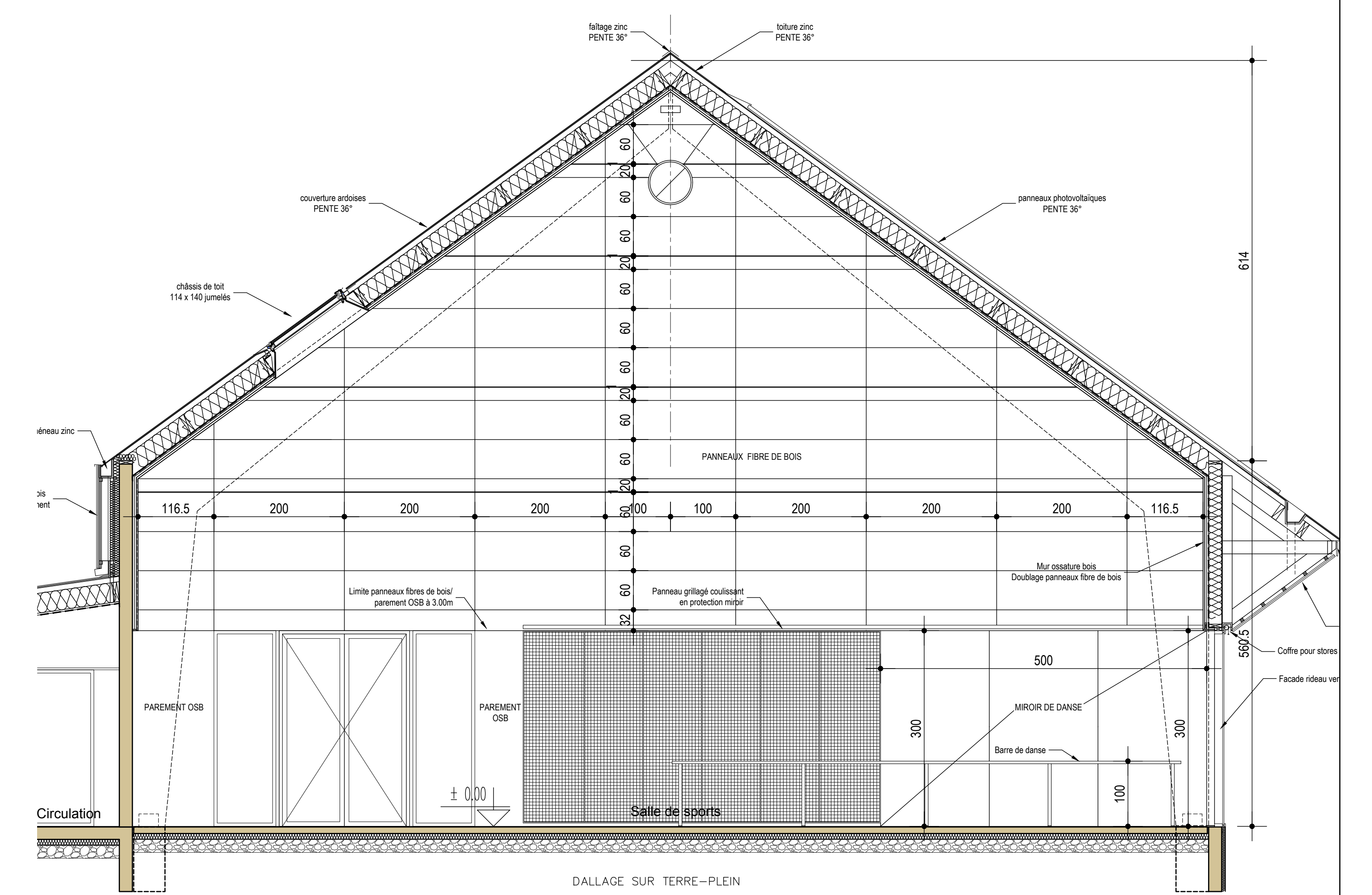
COUPE 7.7 calépinage pignon
