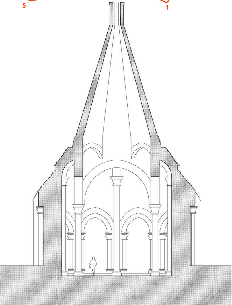
Coupe de principe _ 1/200ème
