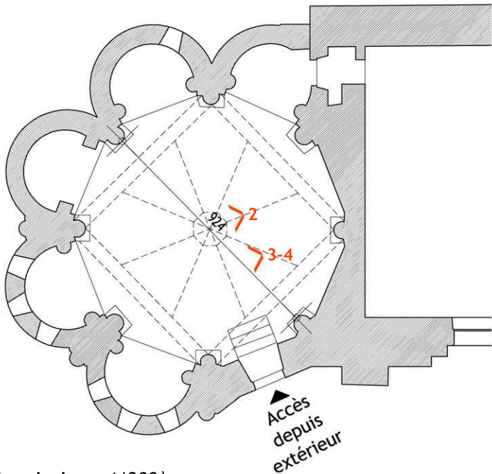
Plan de principe _ 1/200ème
