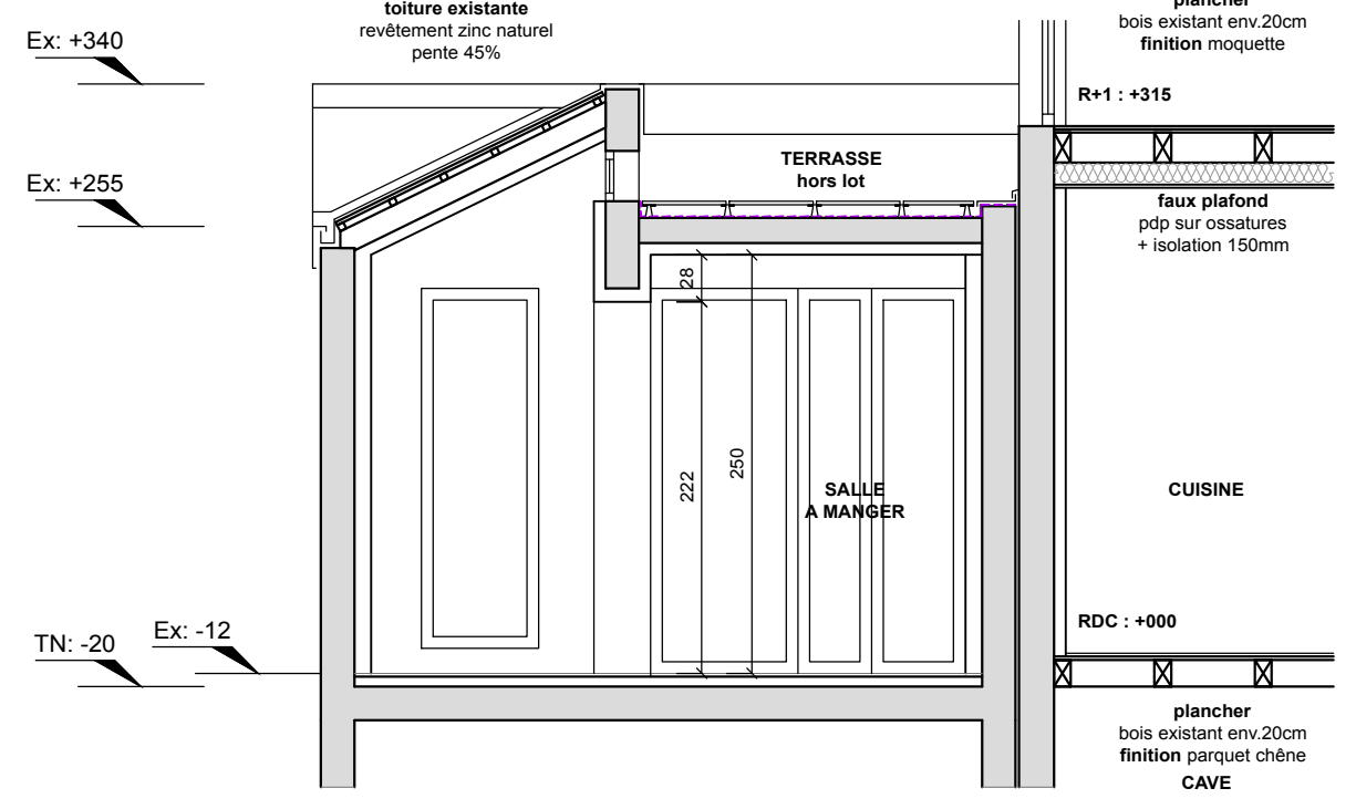
COUPE EXISTANTE
