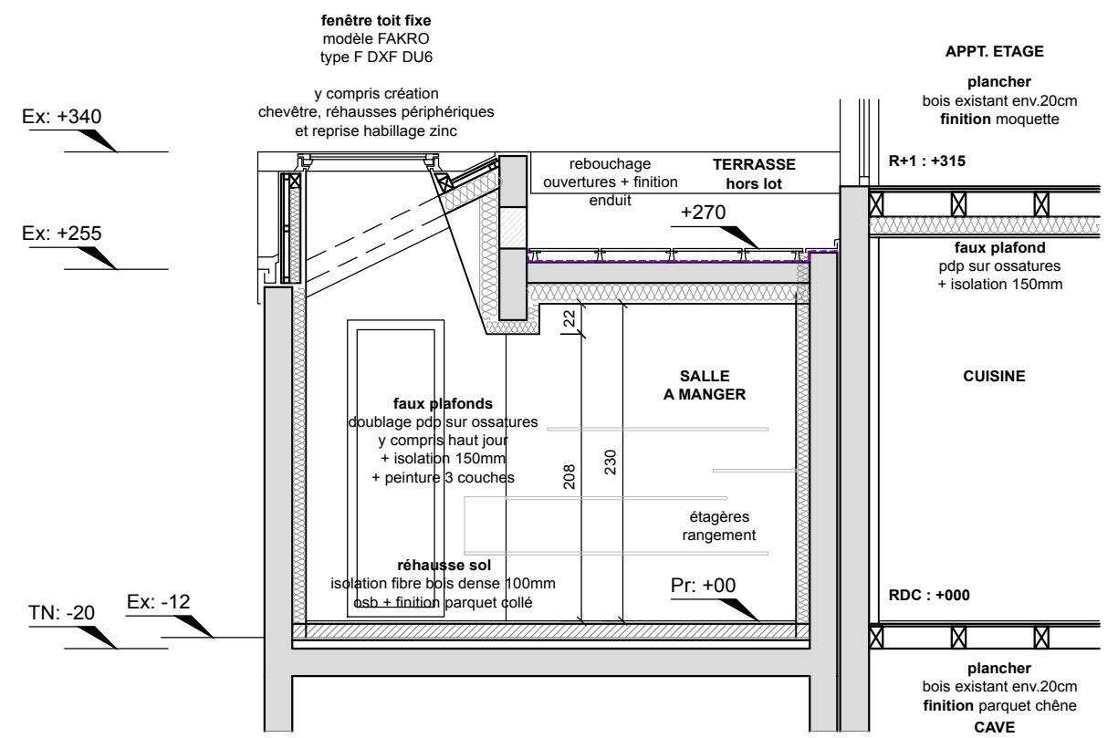
COUPE PROJET
