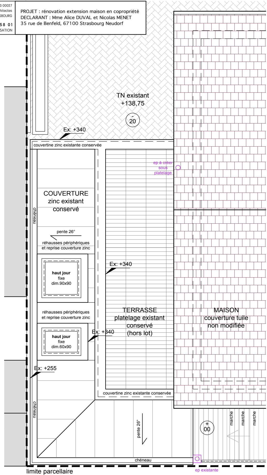
PLAN DE TOITURE PROJET
