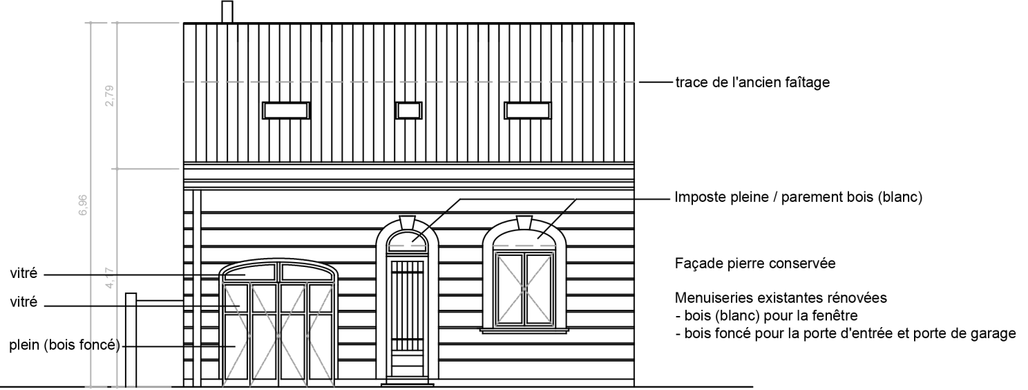
FACADE Nord sur rue
