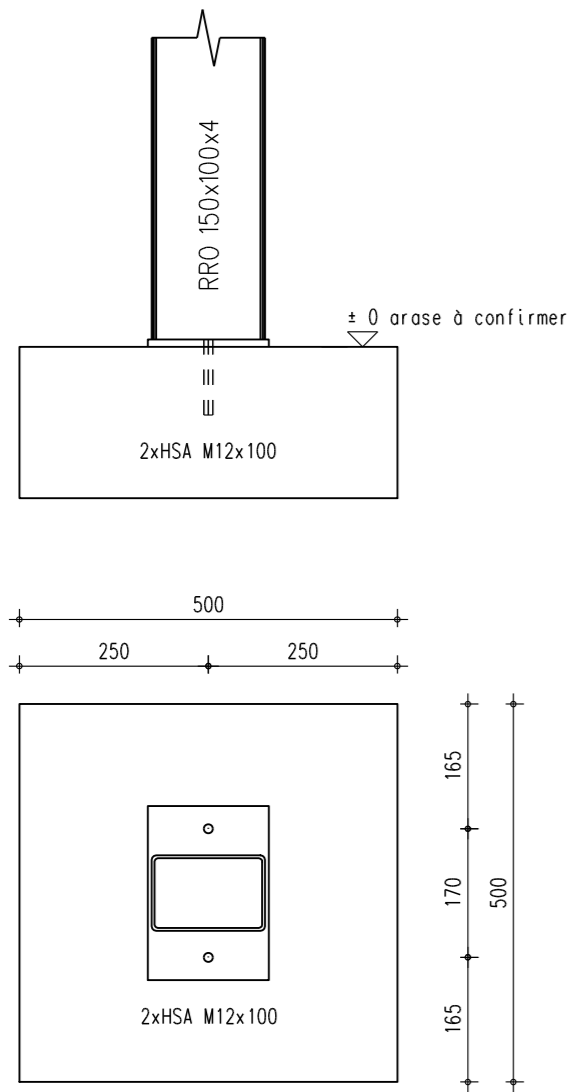
Détail pied de poteau d'entrée Ech. 1:10
