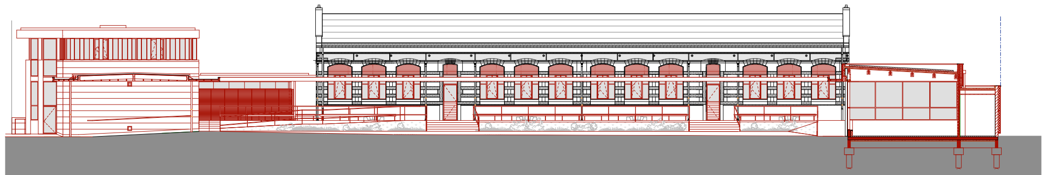
Coupe CC
