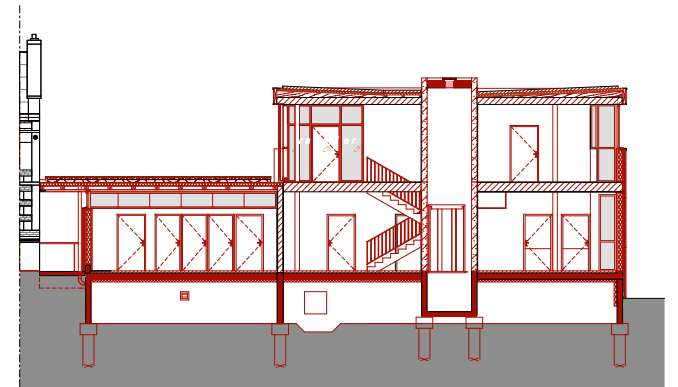
Coupe BB
