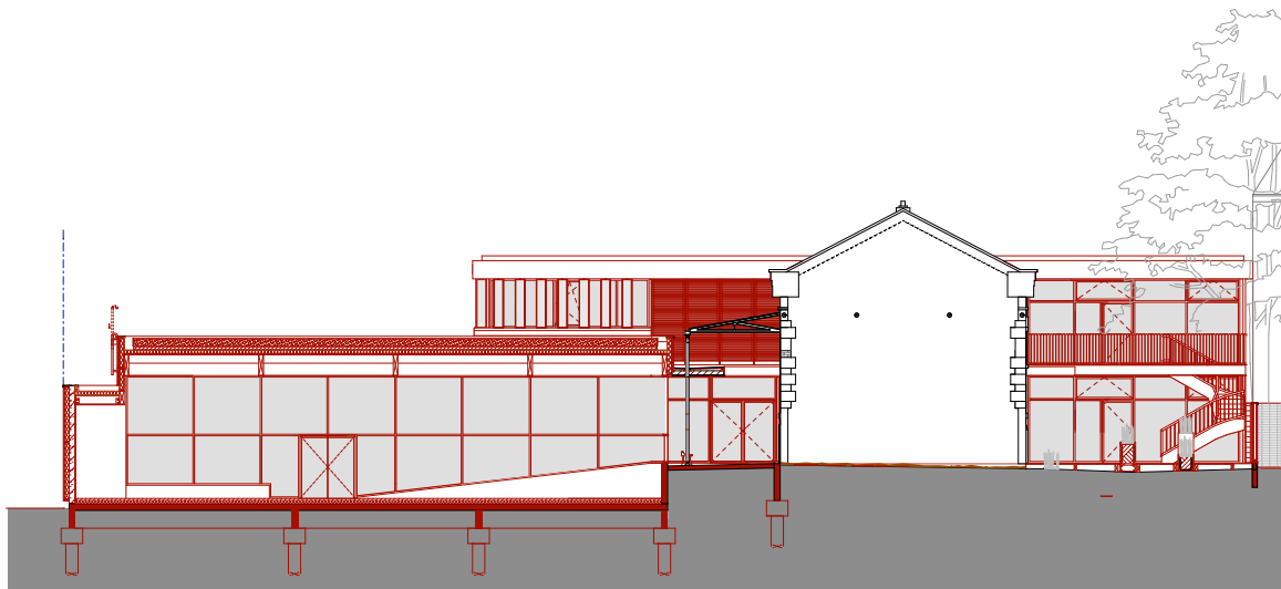
Coupe DD
