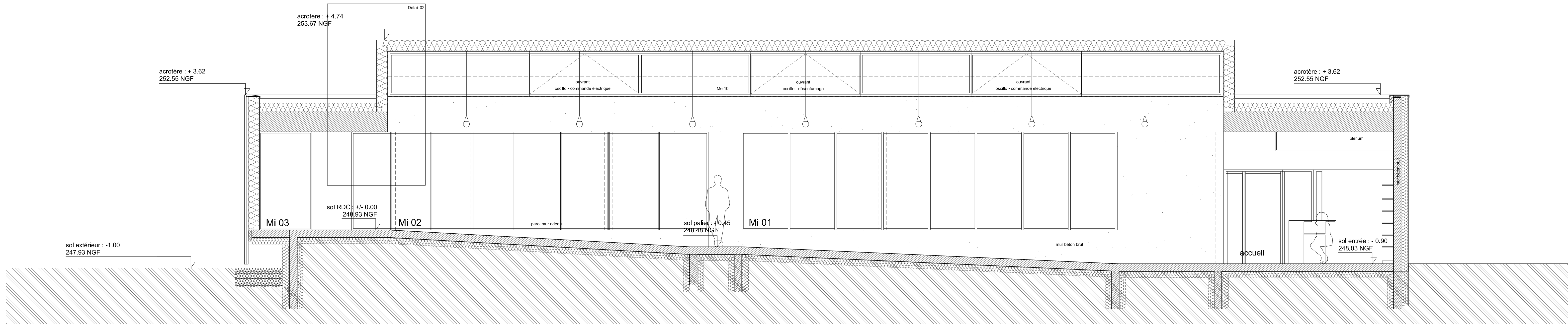
Coupe EE - projet
