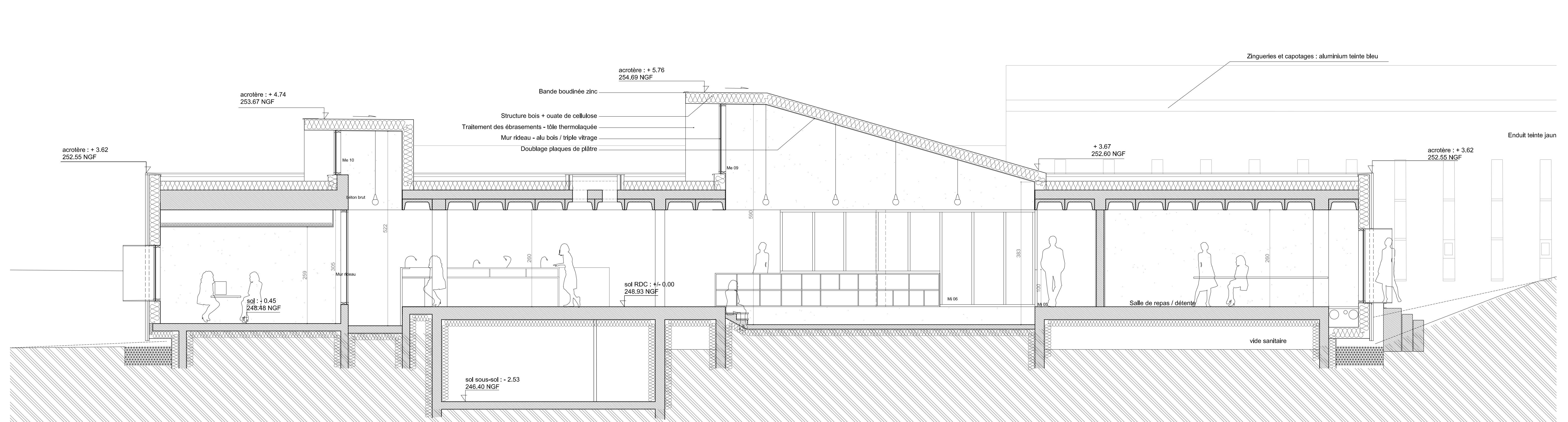
Coupe BB - projet
