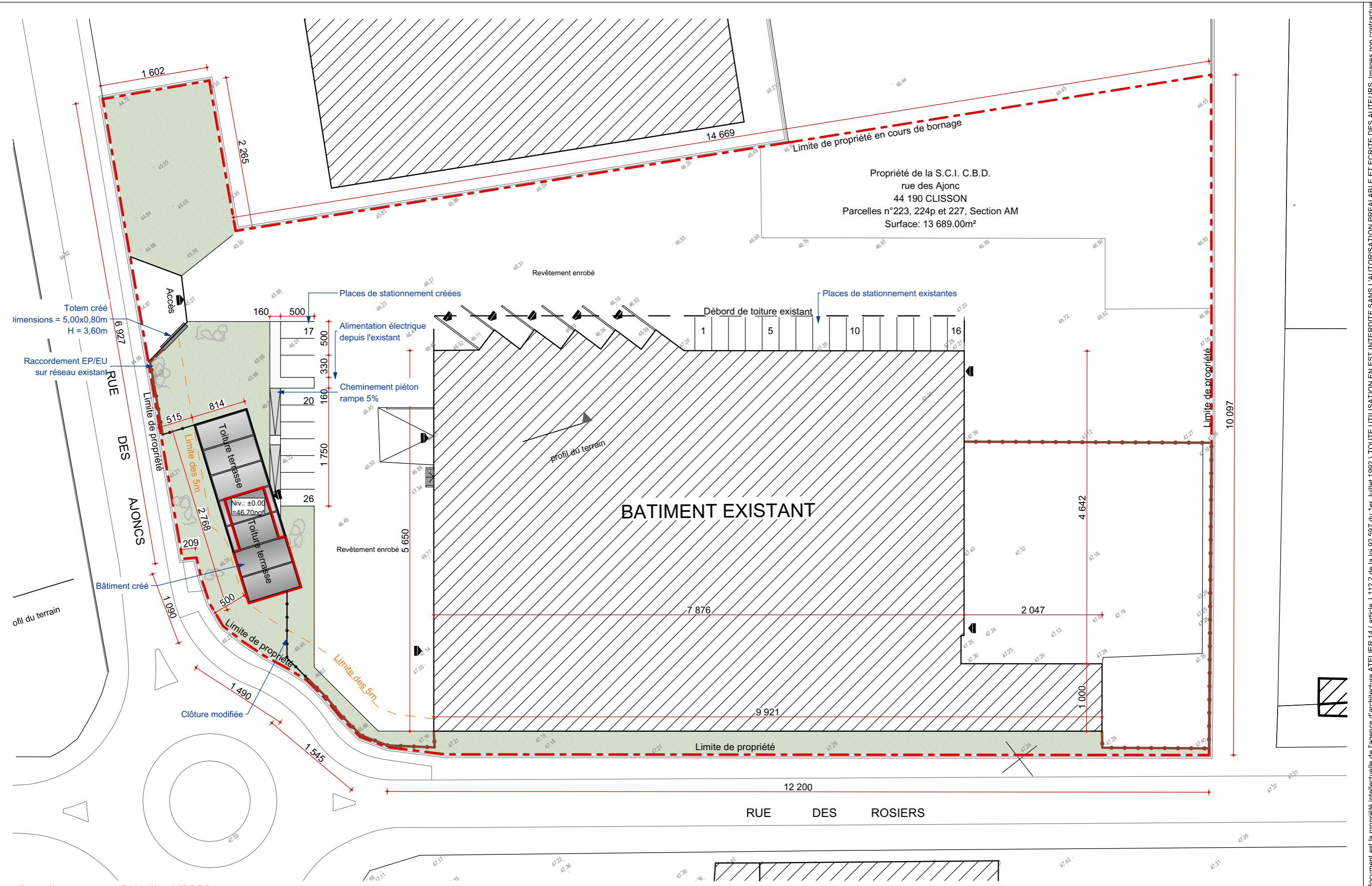
plan de masse - échelle 1/500°
