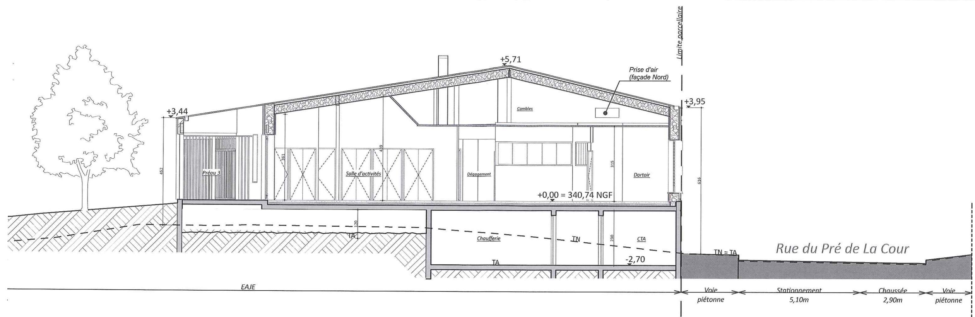
Coupe AA
