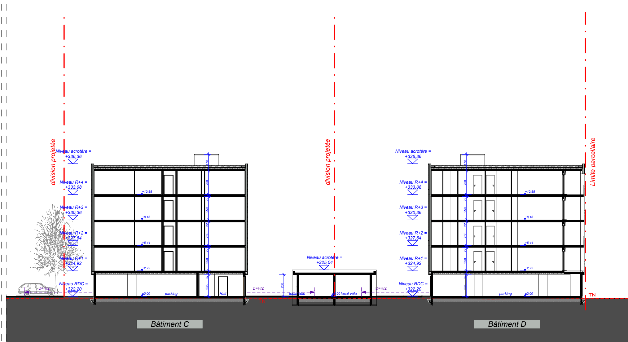
Coupe sur les bâtiments C et D / Ech. : 1/250
