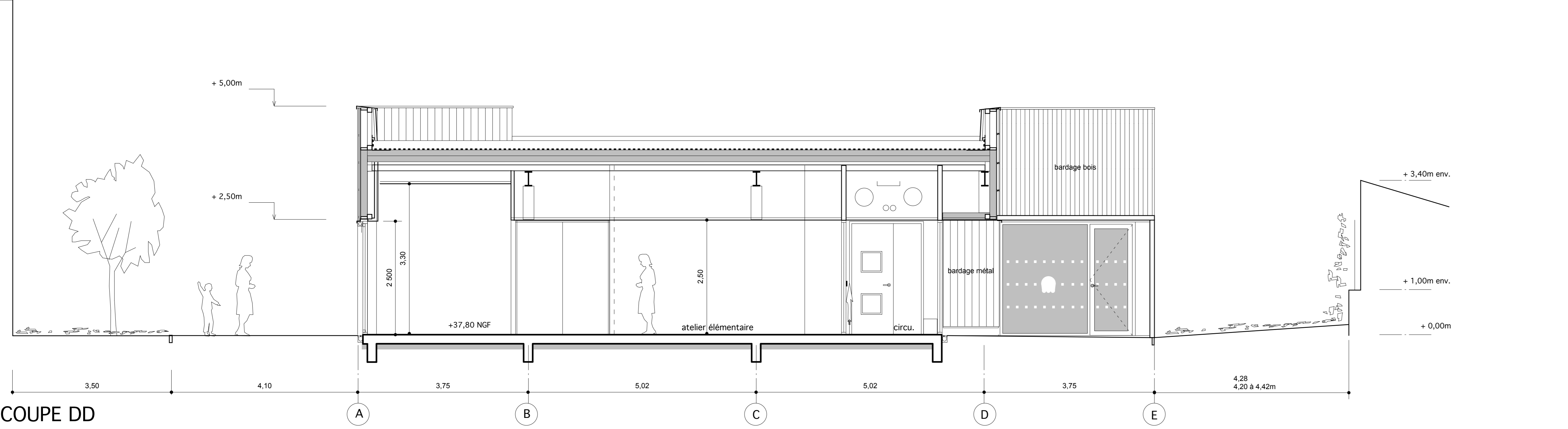
COUPE DD
