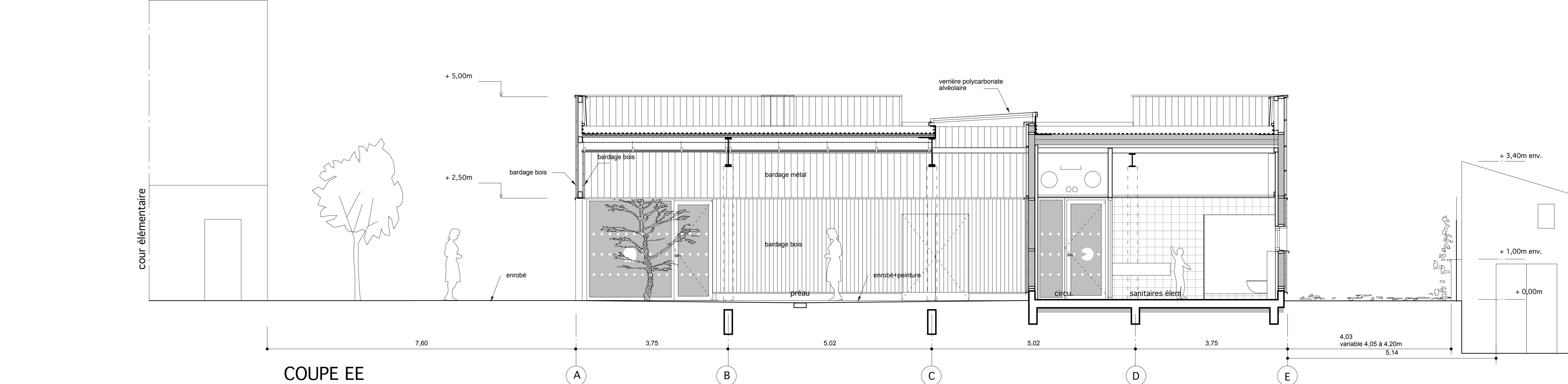
COUPE EE
