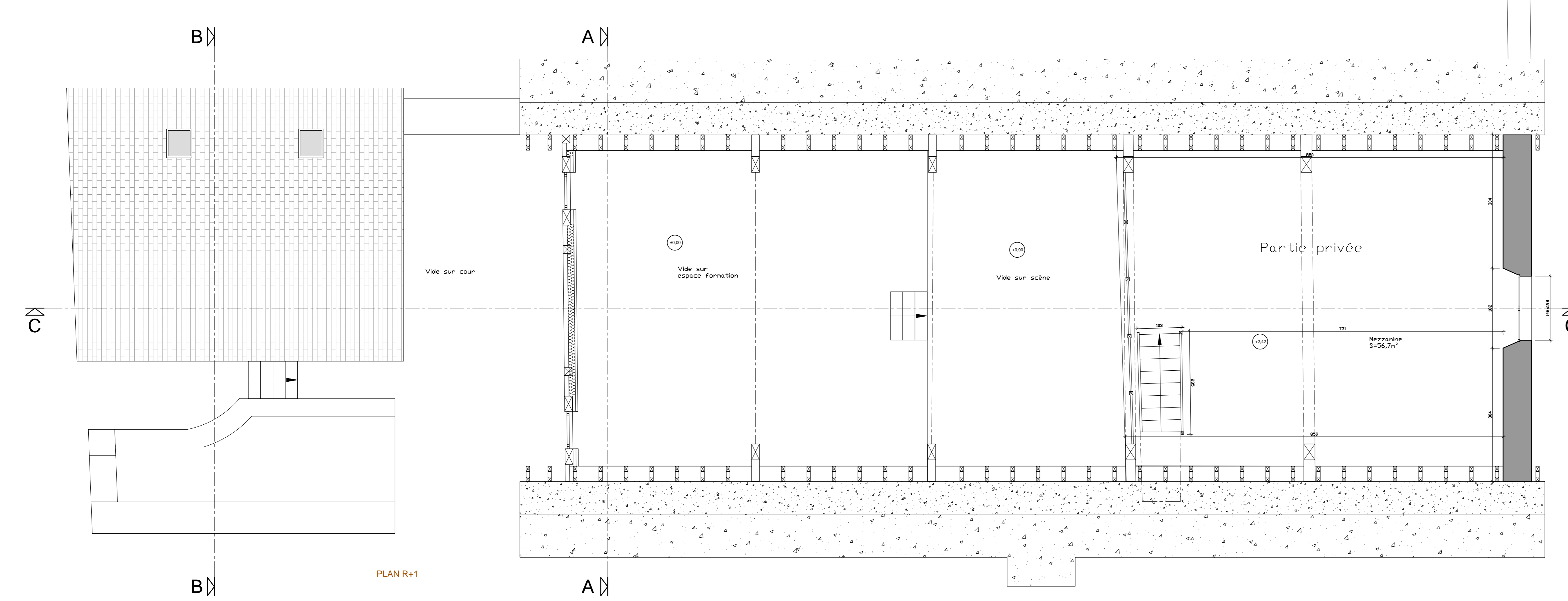
PLAN REZ-DE-CHAUSÉE
