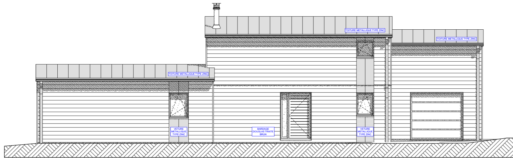
FAÇADE NORD
