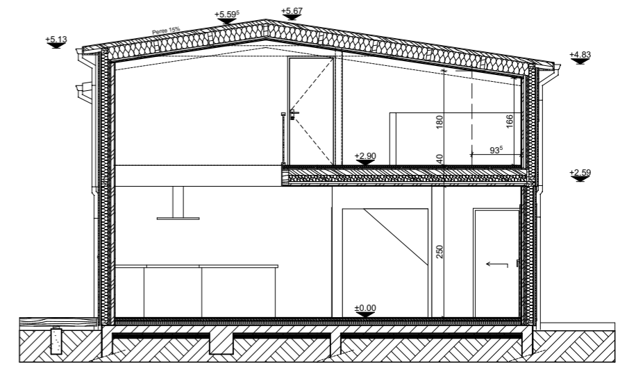
COUPE
