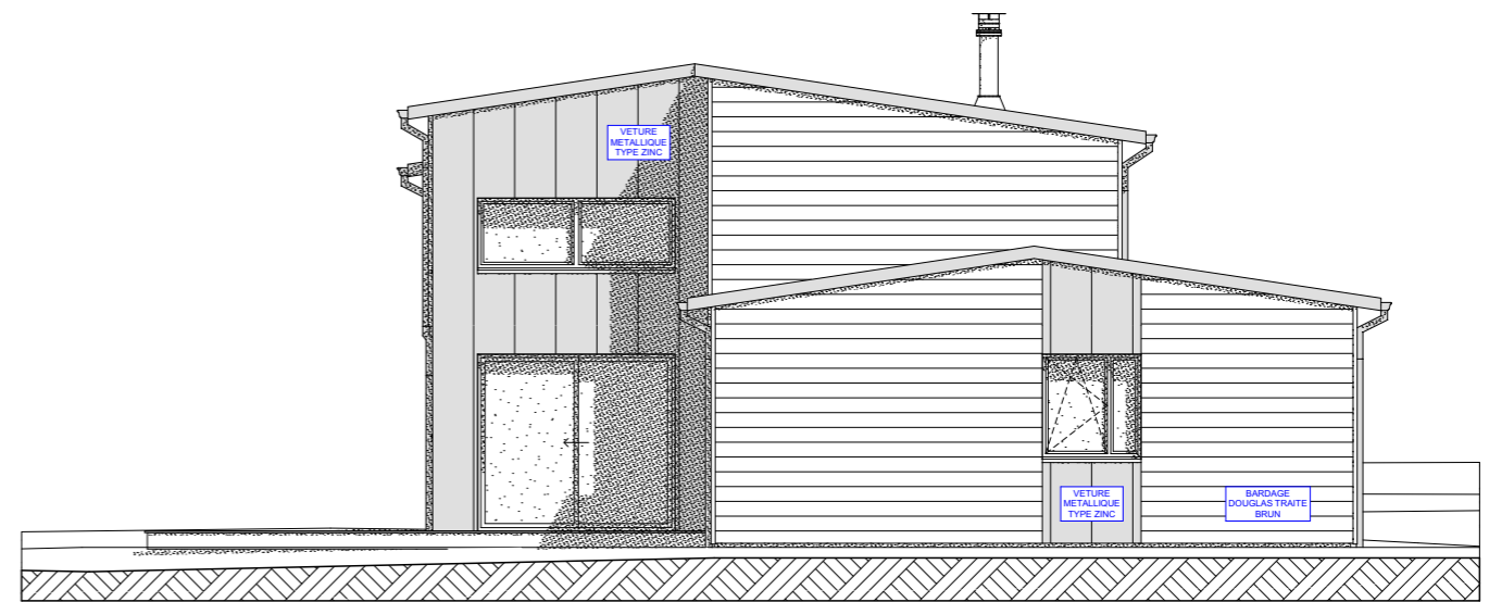
FAÇADE EST
