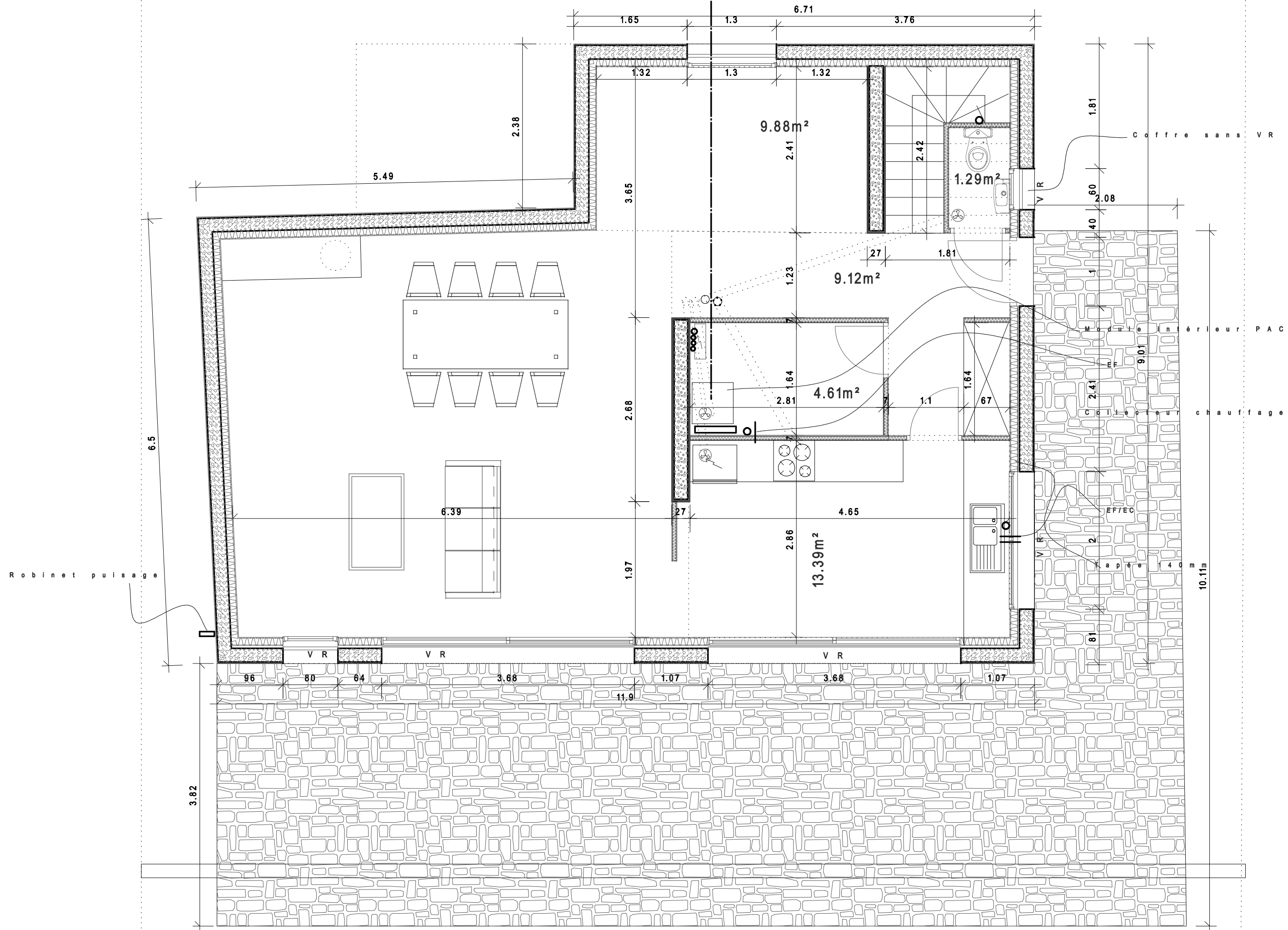
Plan RDJ, ech 1/50eme, le 16 05 17
