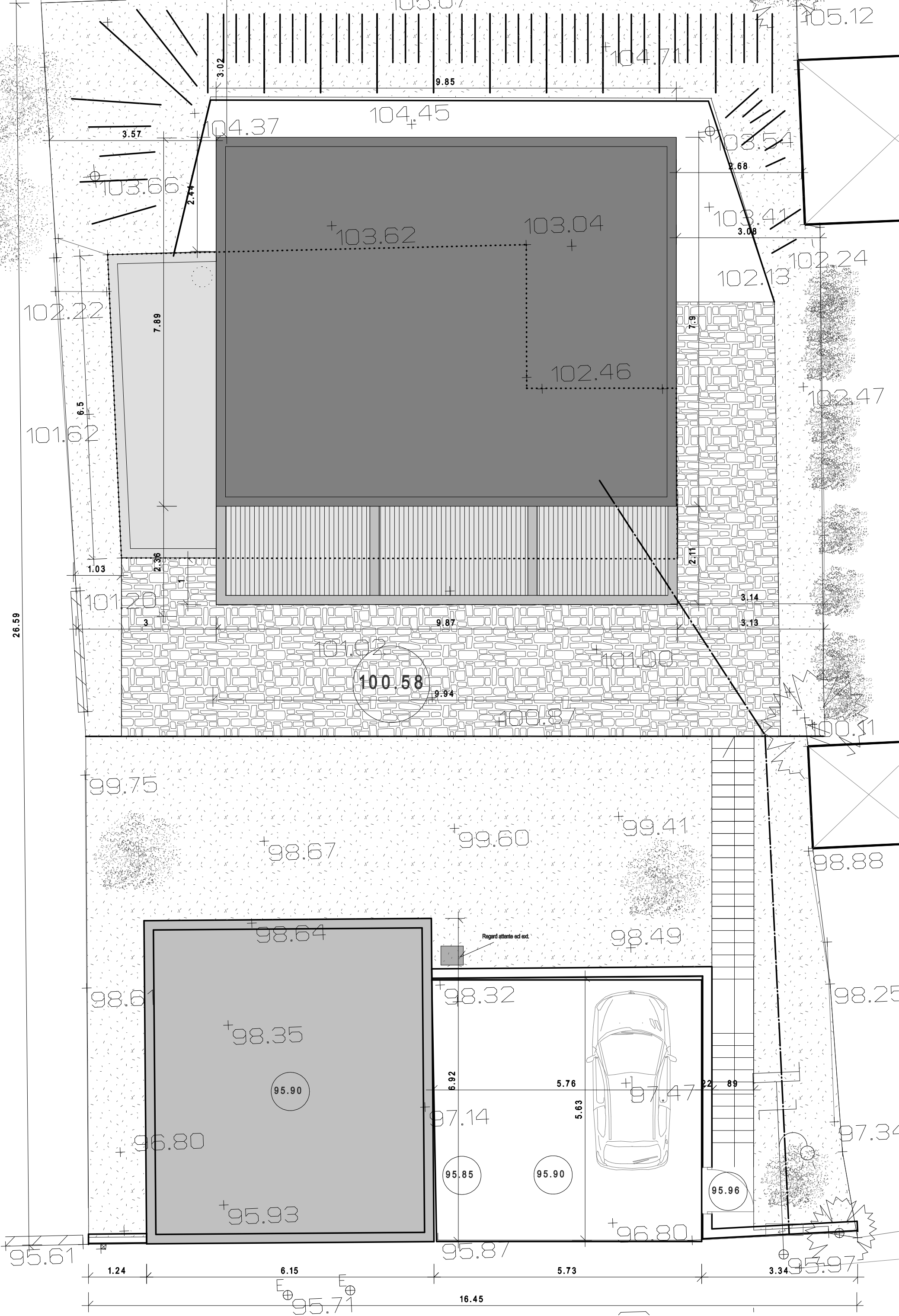
PLAN MASSE, ech 1/70eme, le 16 05 17
