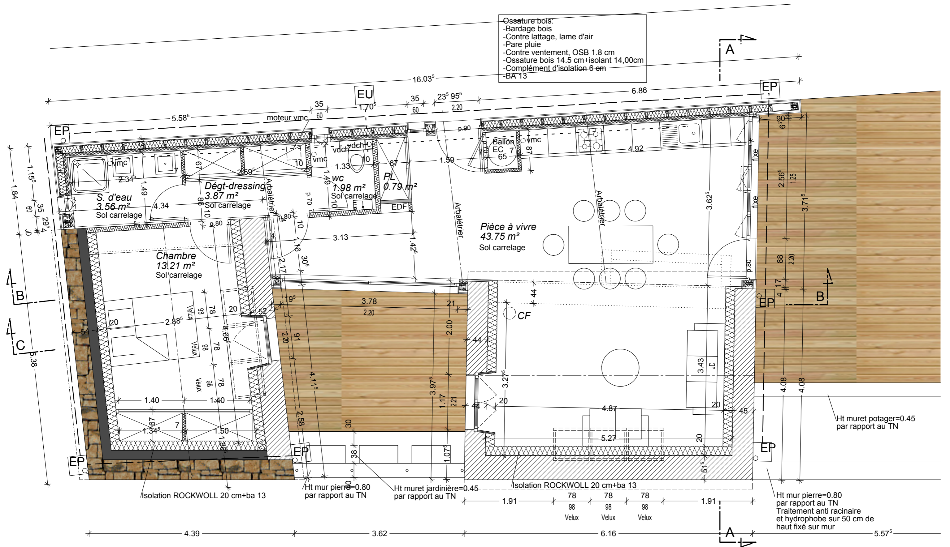
PLAN éch:1/50 Modifié le 11-05-2015: Porte d'entrée+châssis latéral
