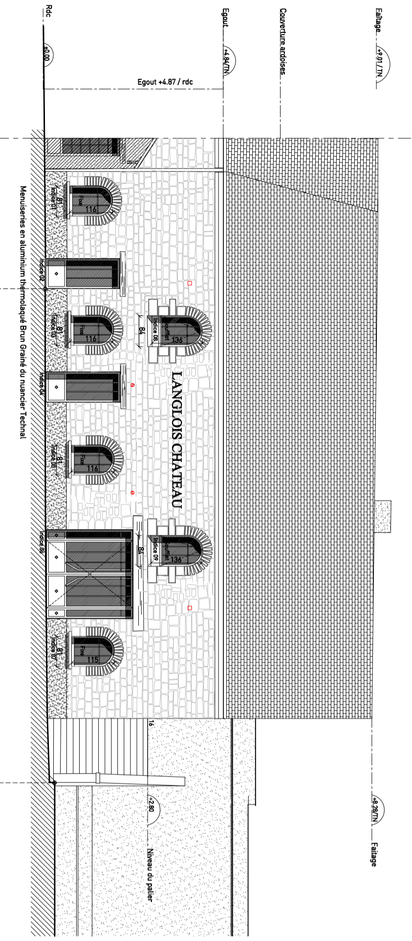
Elévation Est | Etat Futur
