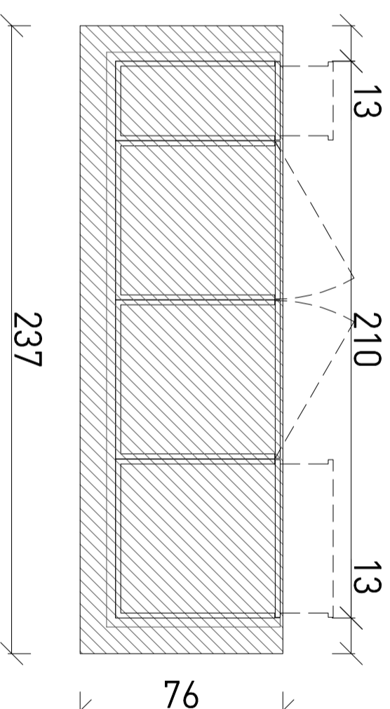
Vue en plan Meuble G I 1/20
