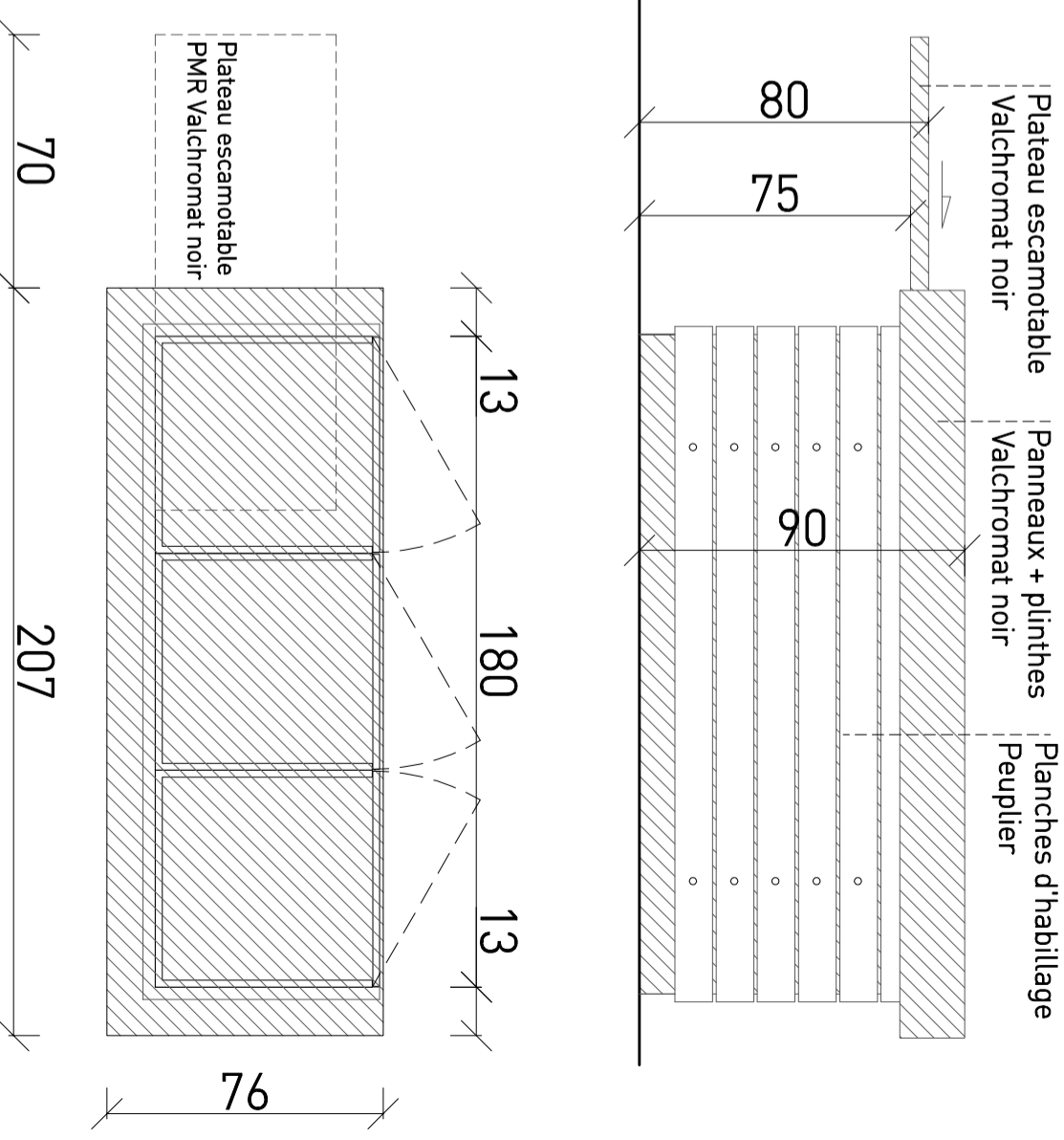
Vue en plan Meuble F I 1/20
