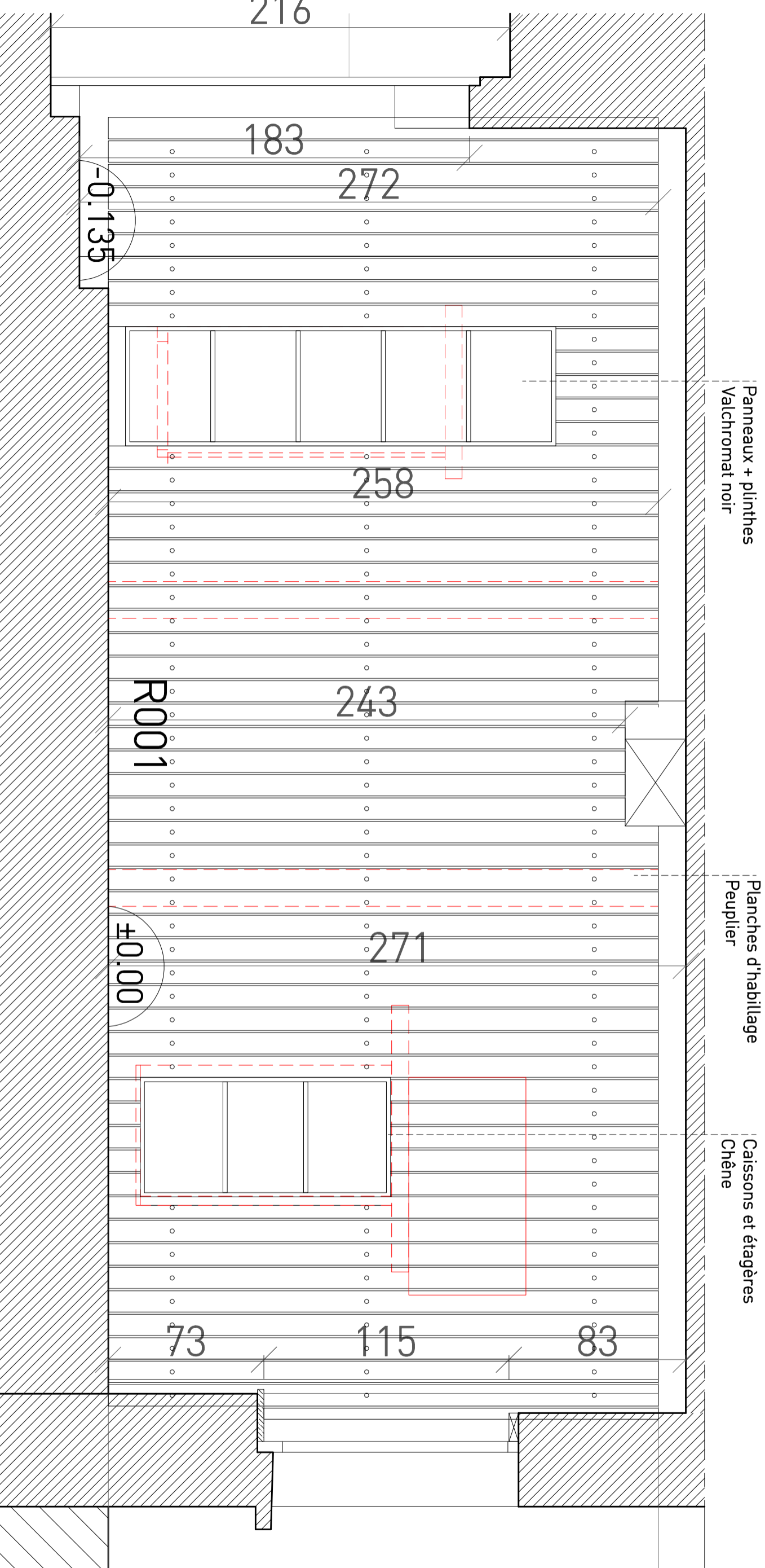
Elevation I - 1/20
