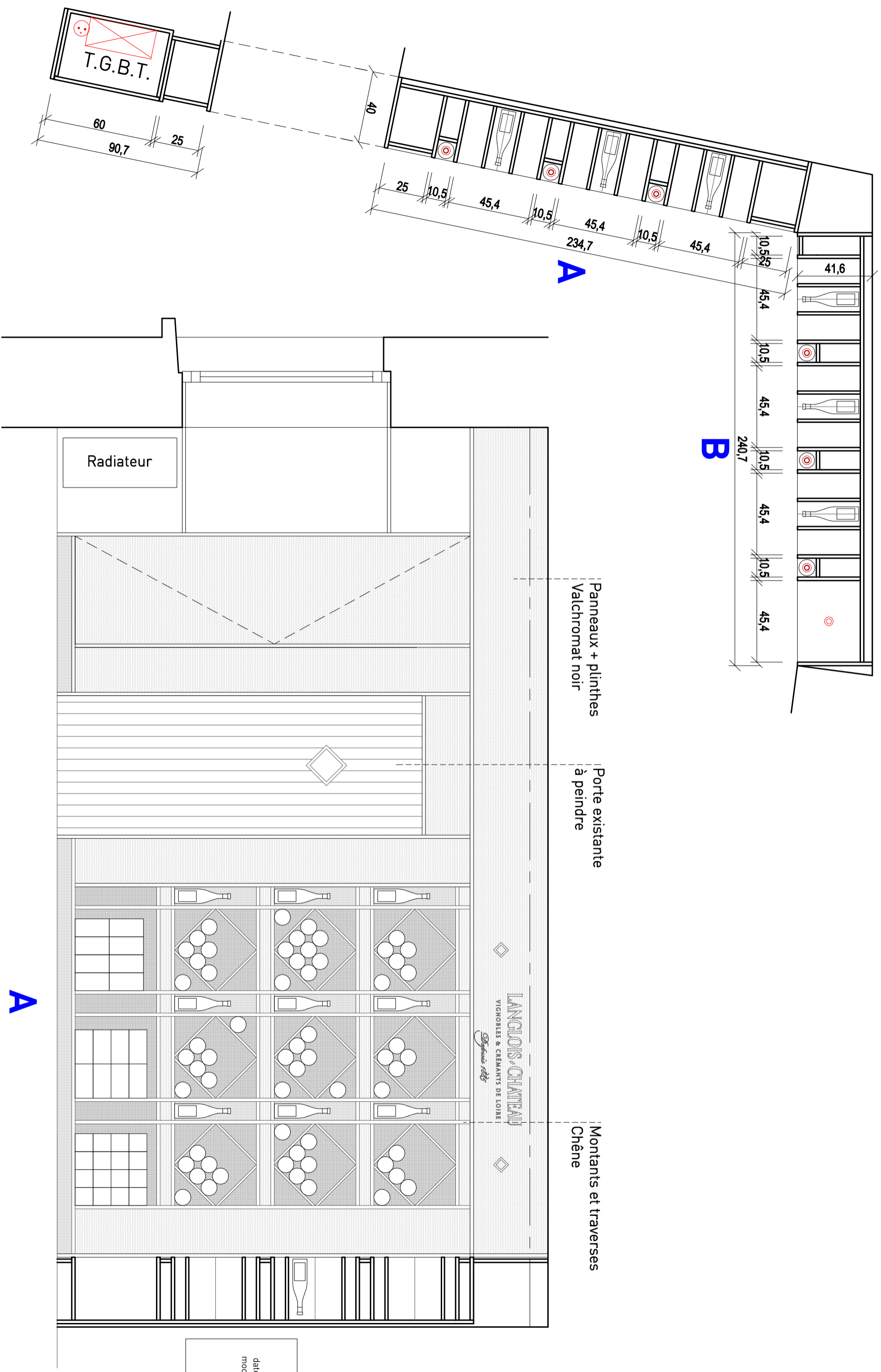
Vue en plan Meuble A & B | 1/20
