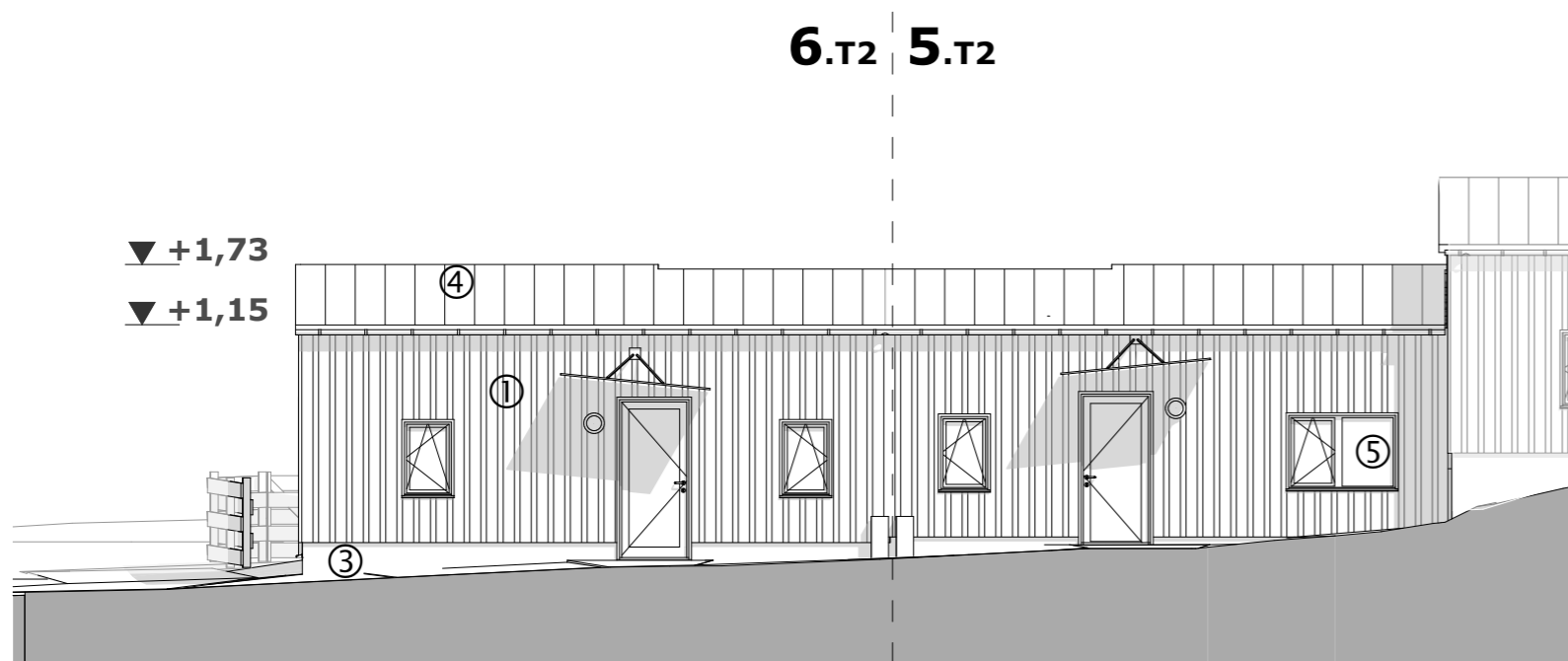
Elévation NORD
