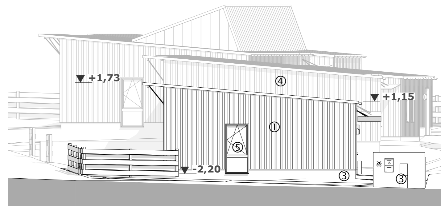
Elévation EST
