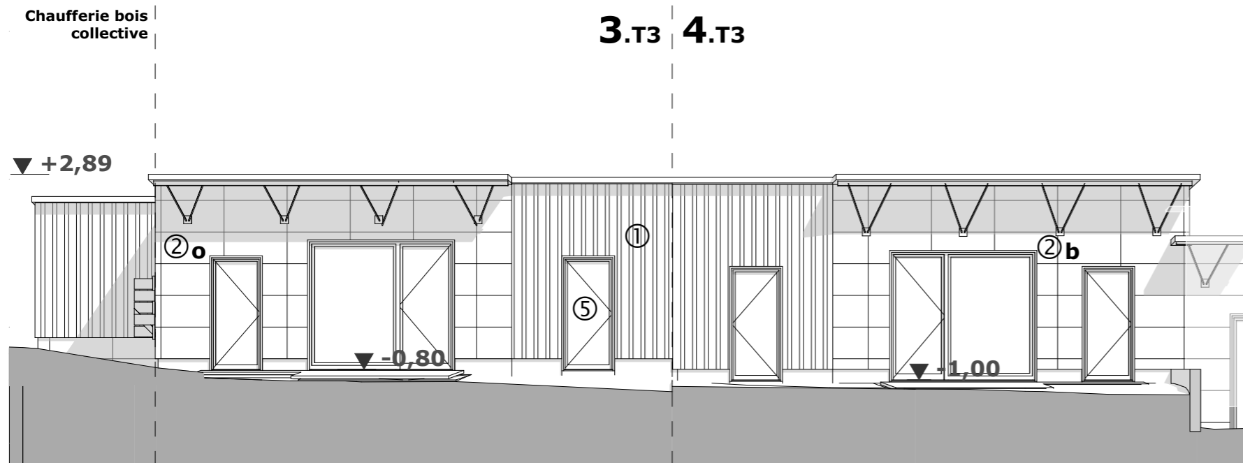
Elévation SUD
