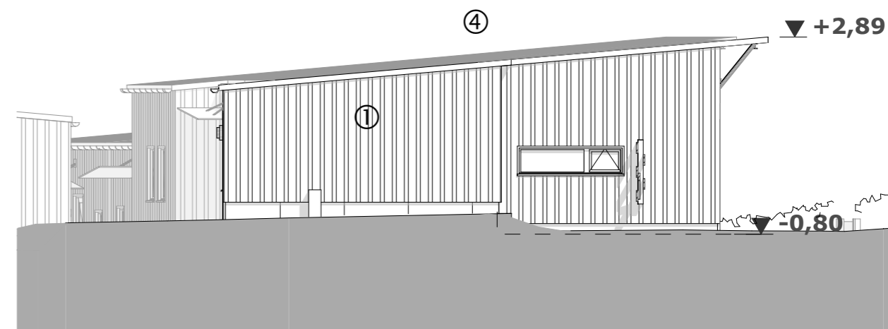
Elévation OUEST
