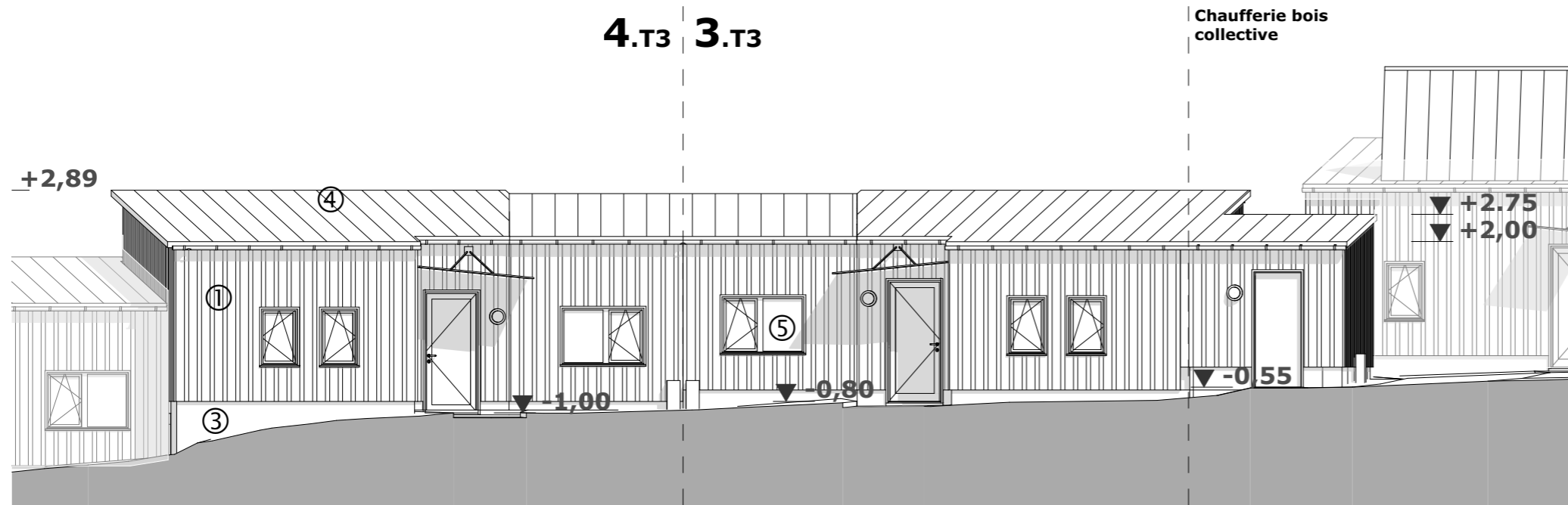
Elévation NORD
