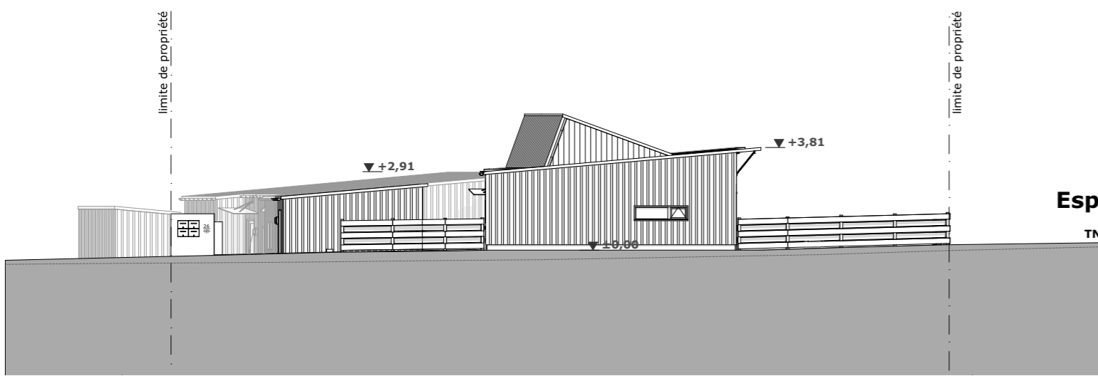
Coupe Nord-Sud / Elévation Ouest
