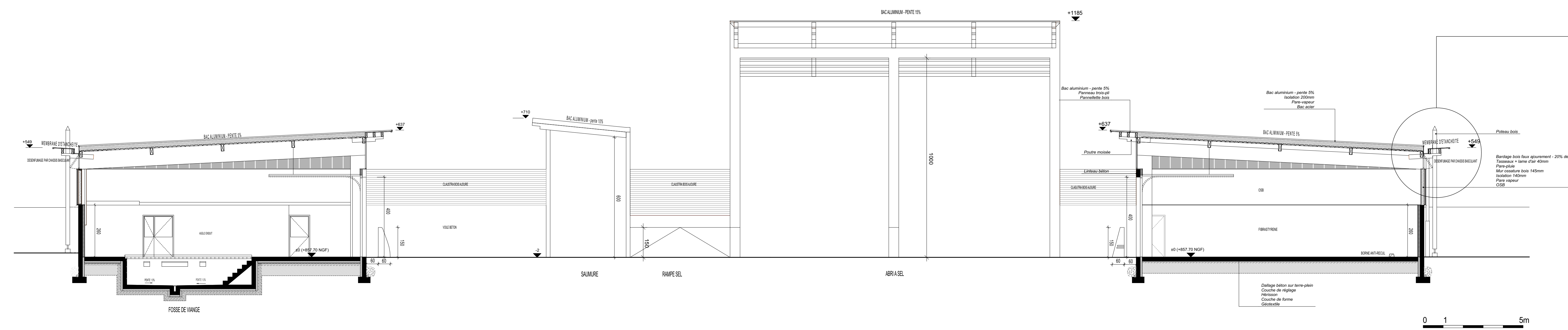
Centre d'Exploitation et d'Intervention du Puy en Velay Coupe CC sur les garages, la cour intérieure et la fosse de vidange Echelle 1 : 100
