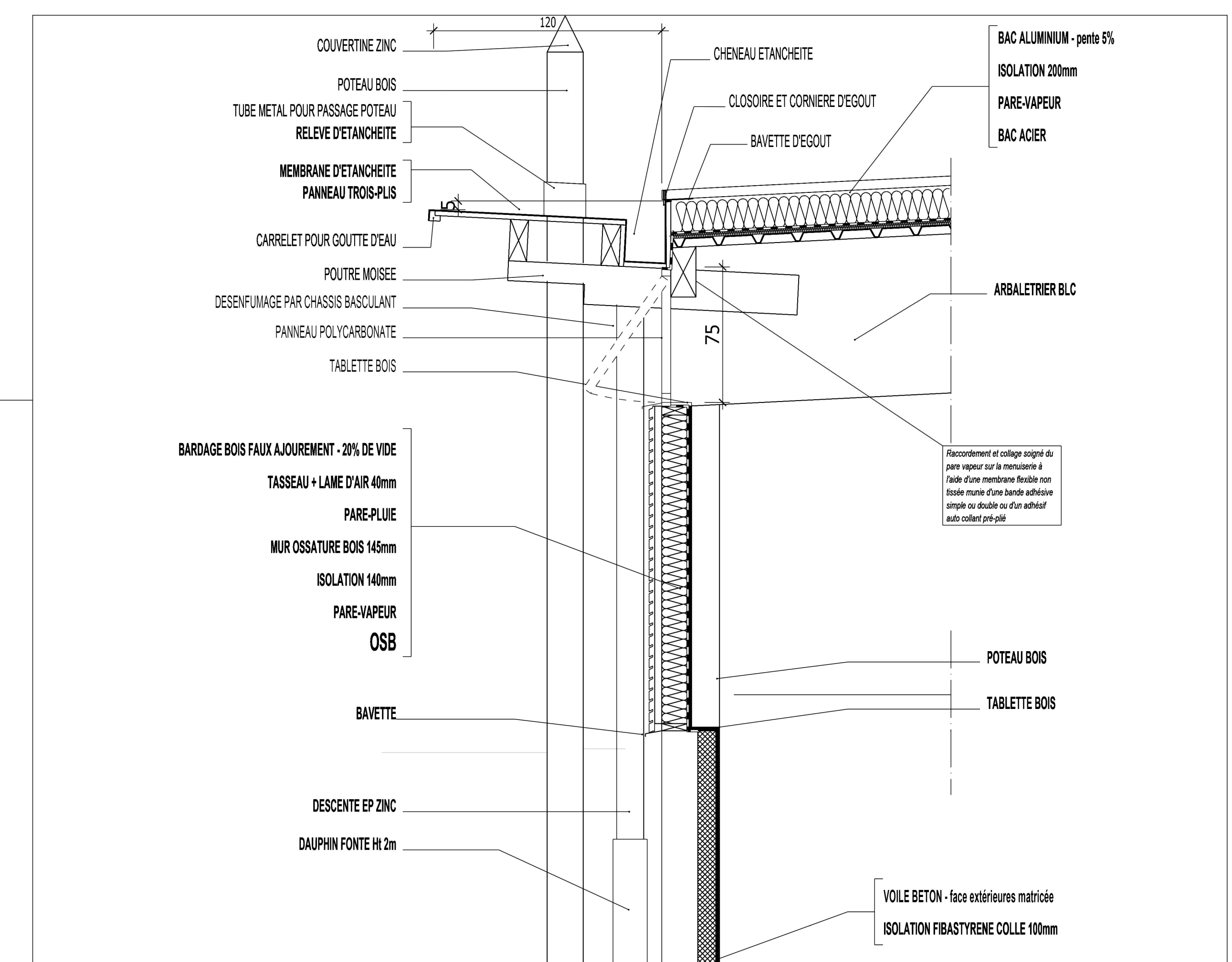
Centre d'Exploitation et d'Intervention du Puy en Velay Détail constructif sur la liaison mur-toiture Echelle 1 : 20
