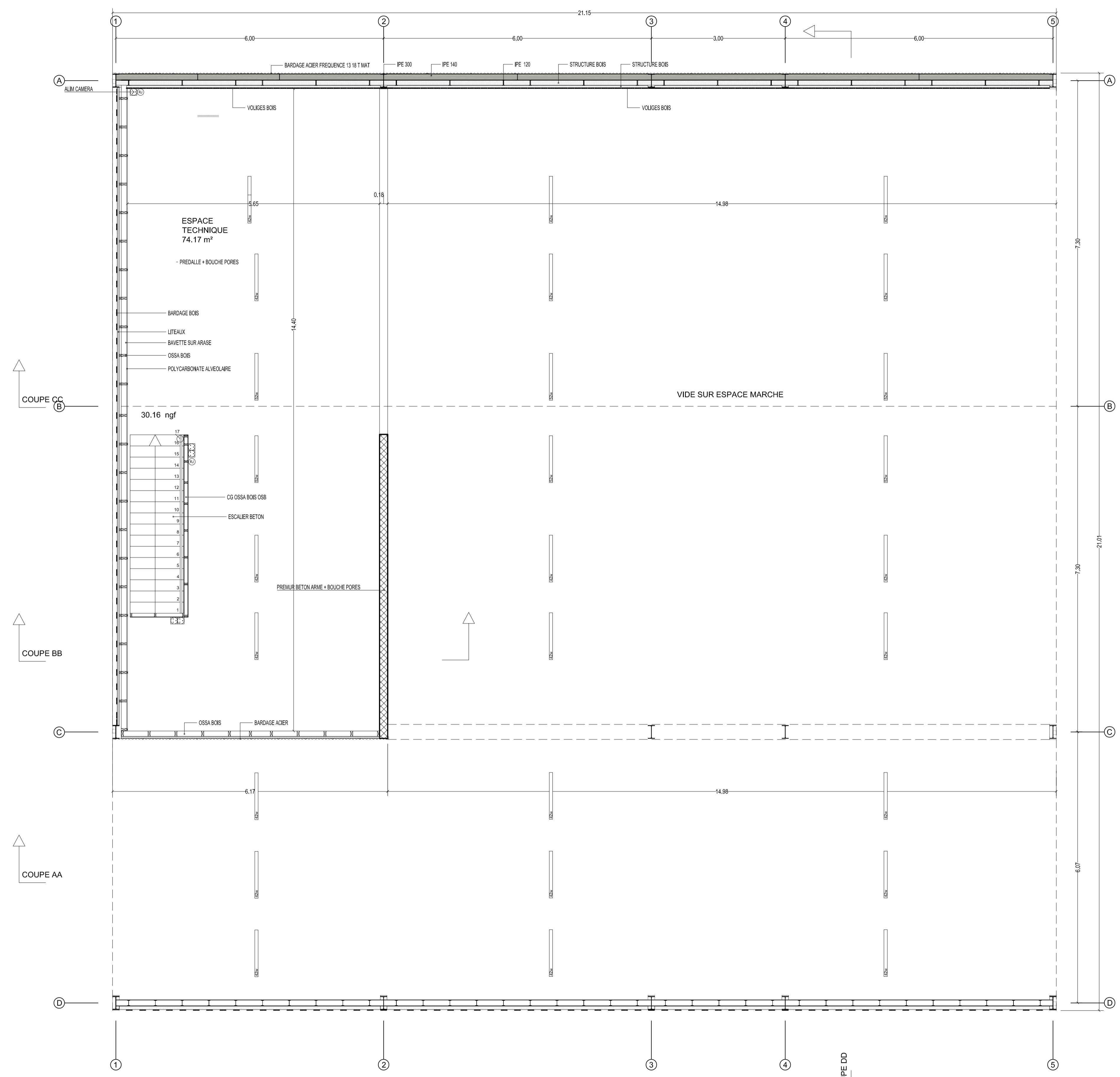
Plan niveau mezzanine 1/50è
