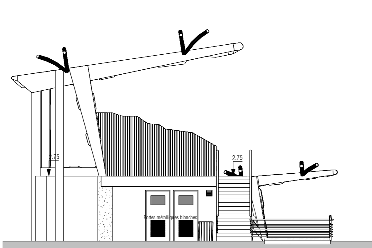
PROJET-FACADE EST Ech.: 1:100
