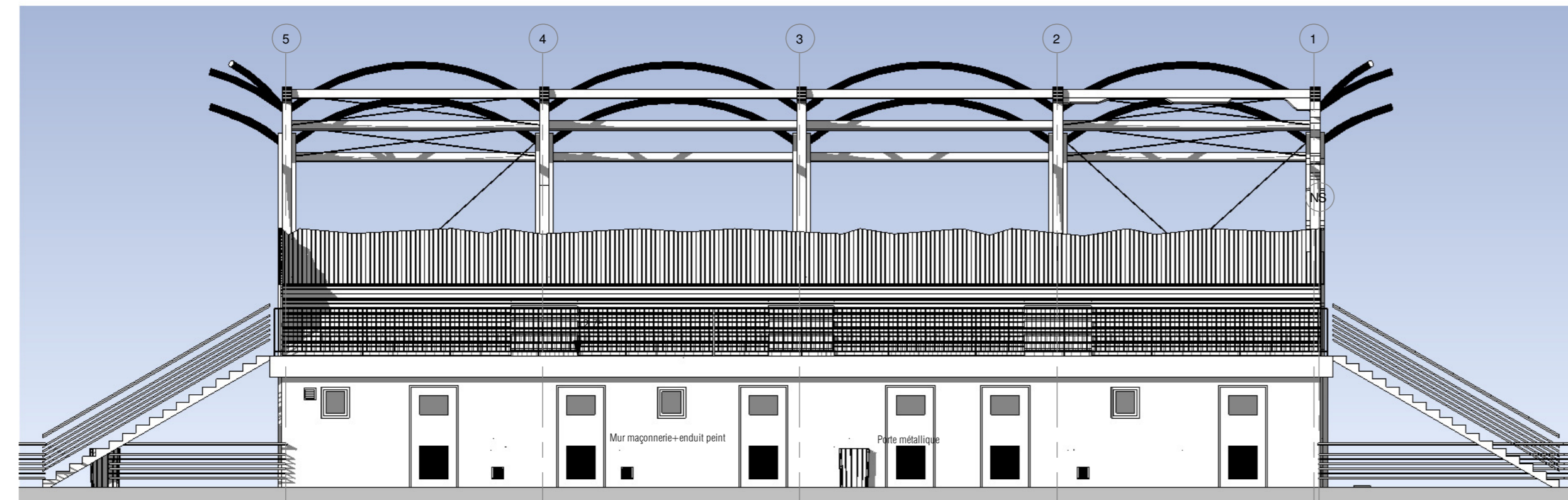
PROJET-FACADE NORD Ech.: 1:100
