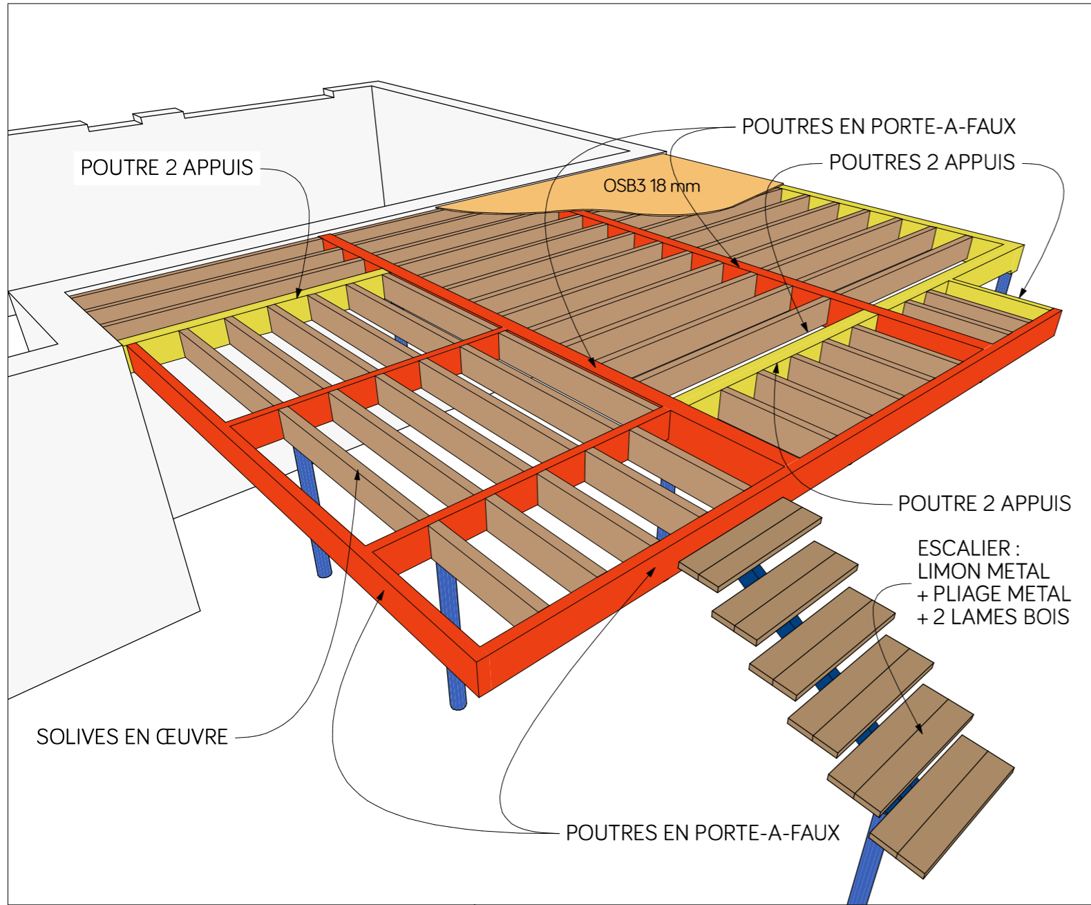
principe ossature plancher bas | vue 3 D
