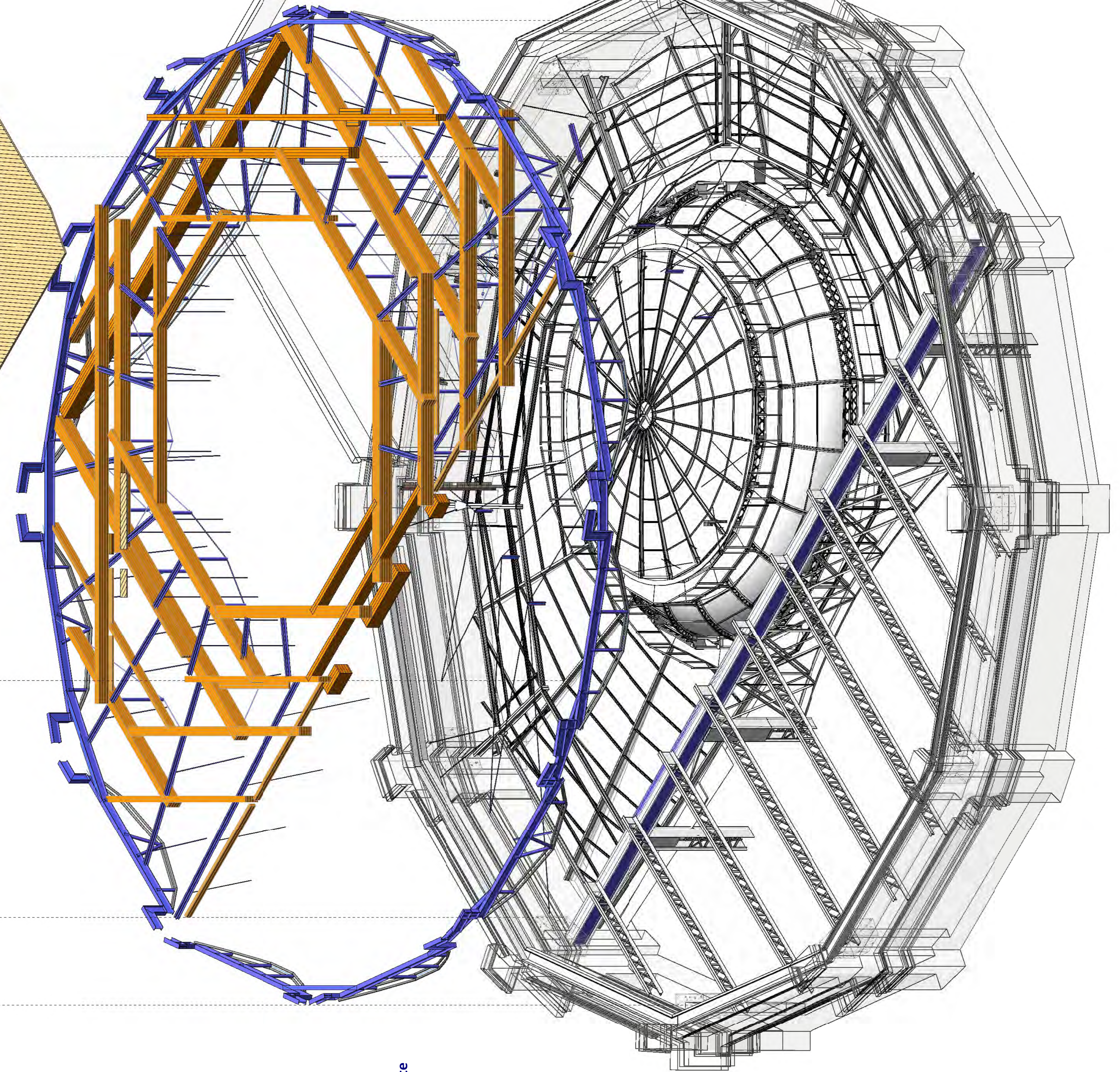
3.- Ceinture périphérique d'appuis + Poutrason en bois pour reprise des plafonds de la Grande Salle
