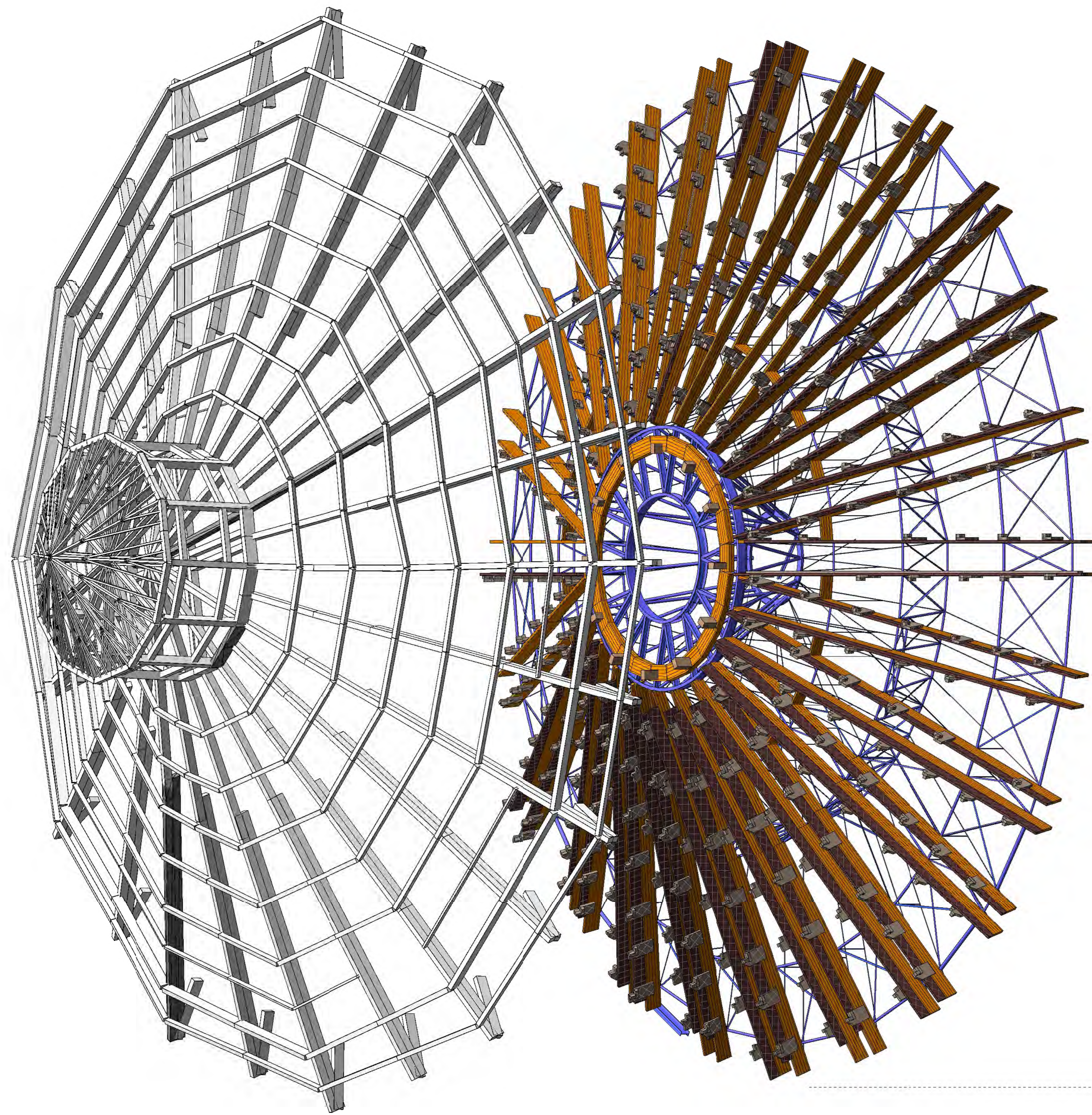
8.- Déconstruction des éléments rendus inutiles sur la charpente de la couverture existante
