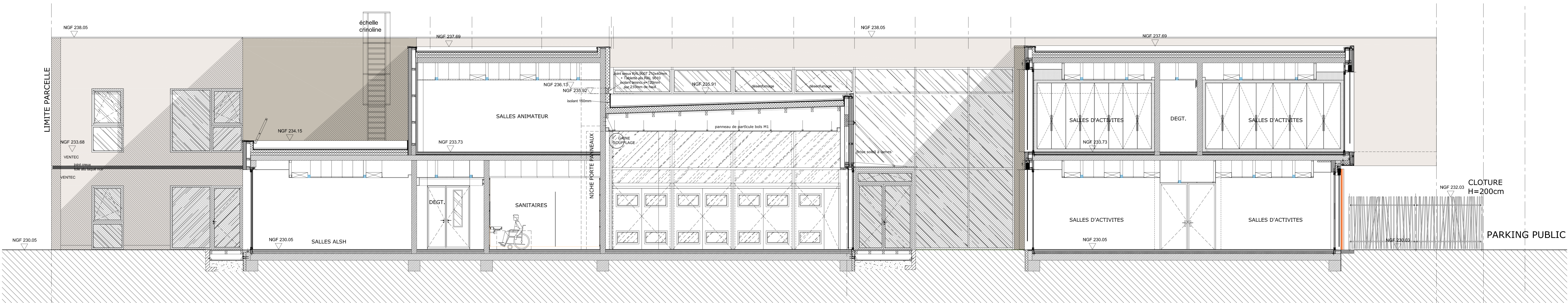
COUPE 3-3
