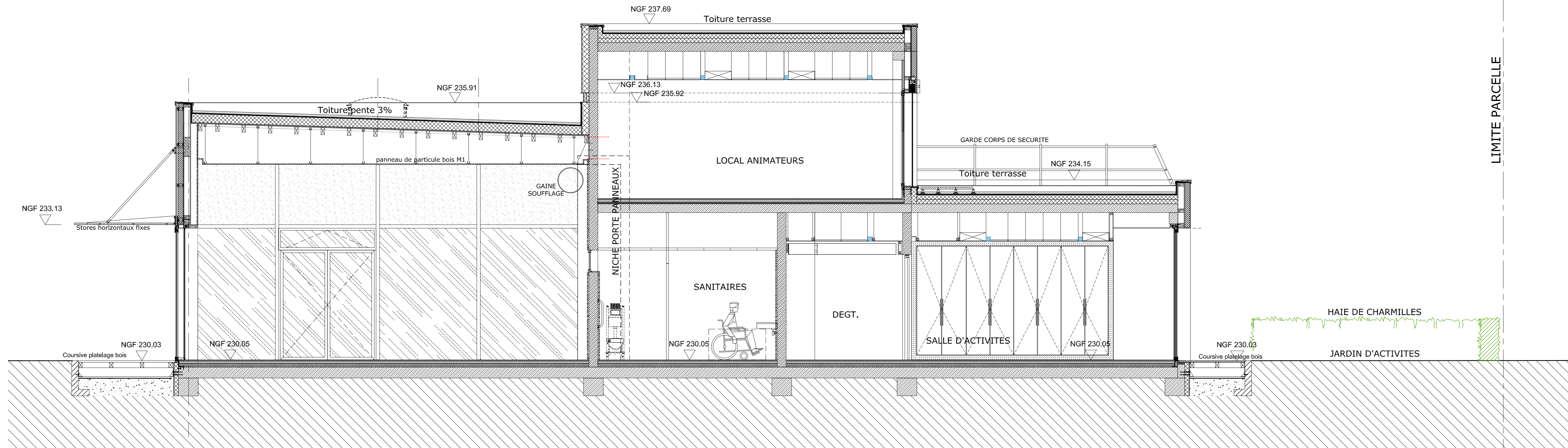
COUPE 2-2
