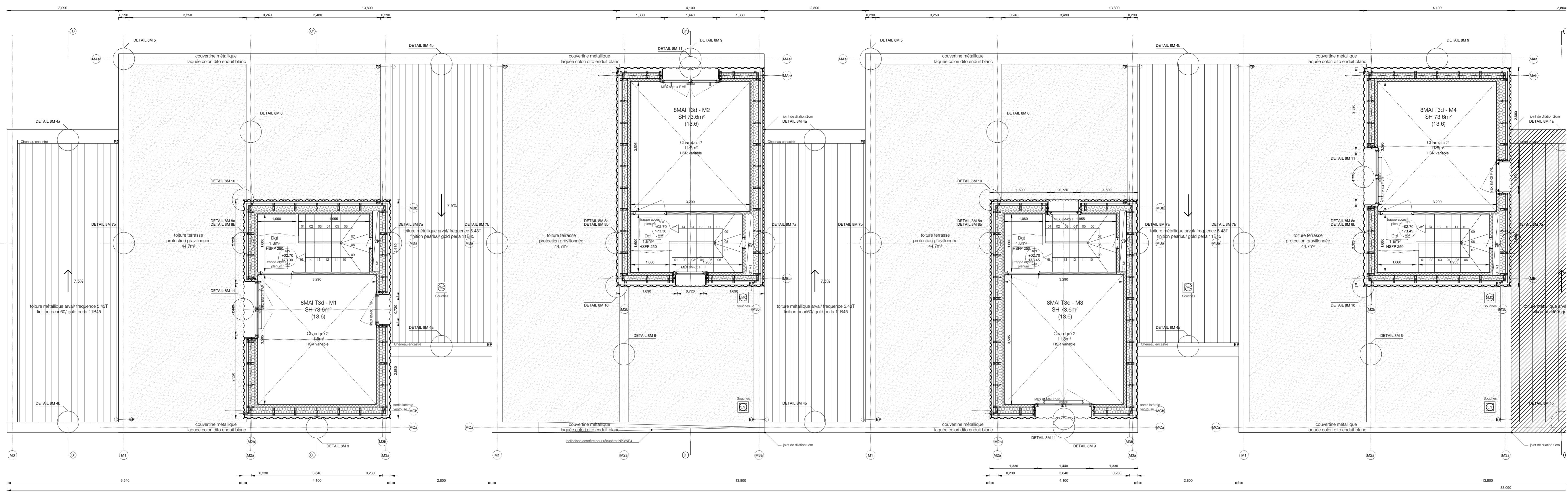
8 MAI M1 à M4 (T3) PLAN R+1 - échelle 1/50e
