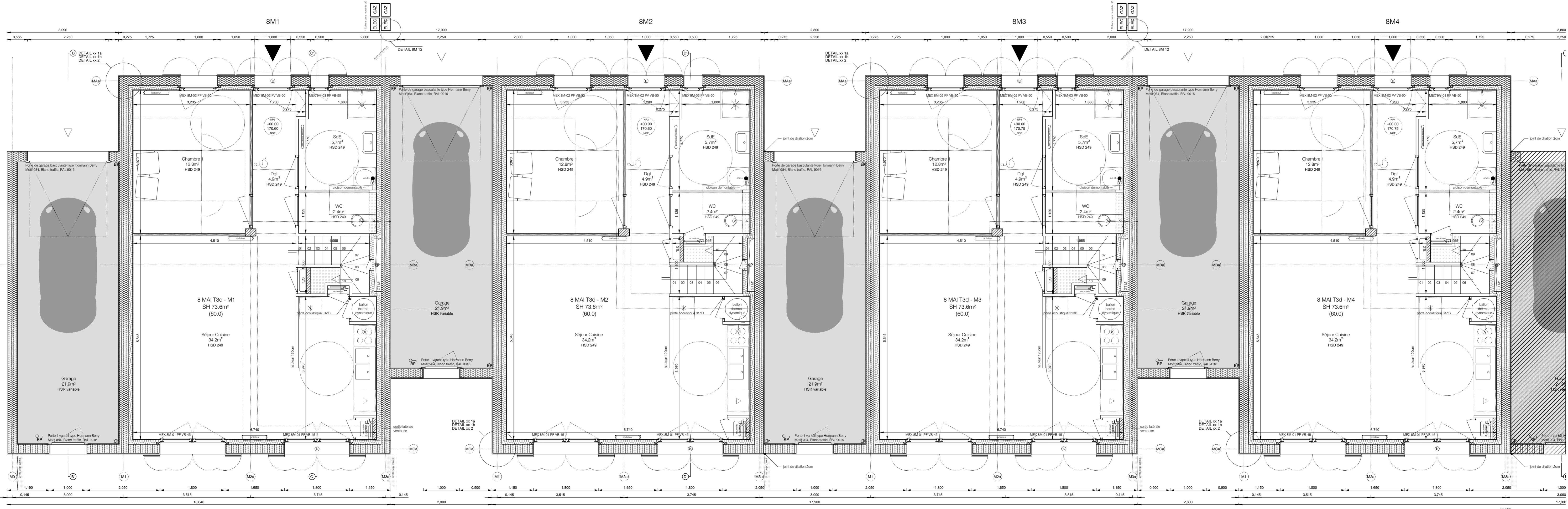
8 MAI M1 à M4 (T3) PLAN DE RdC - échelle 1/50e
